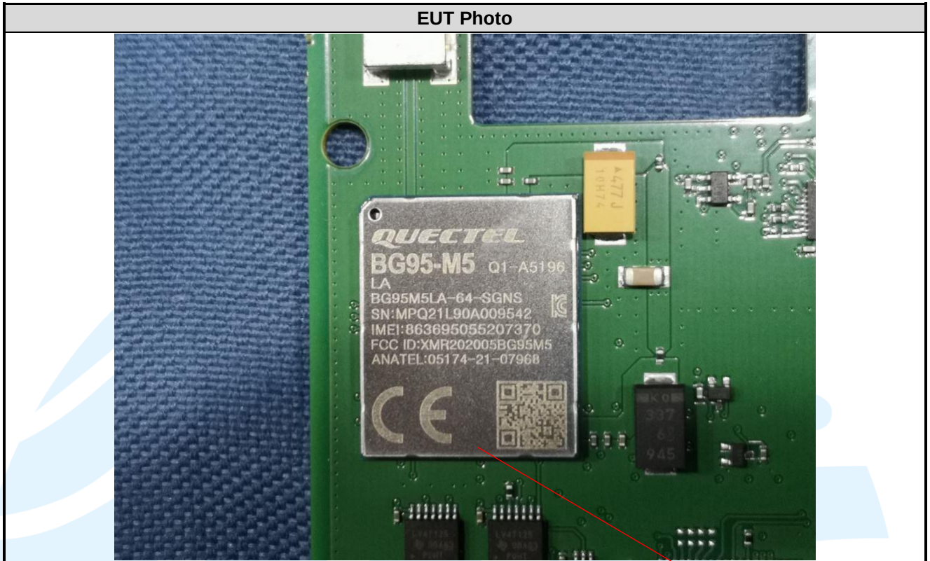
LTE Module
