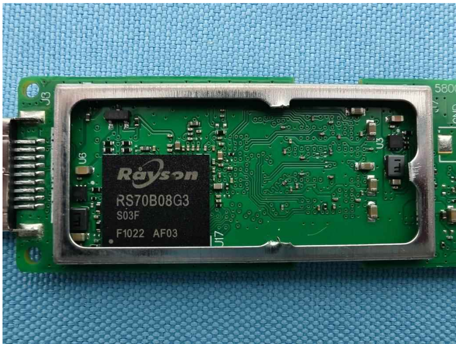
BT&WiFi-ANT1
