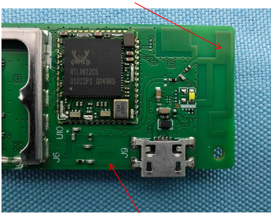
BT&WiFi-ANT1
