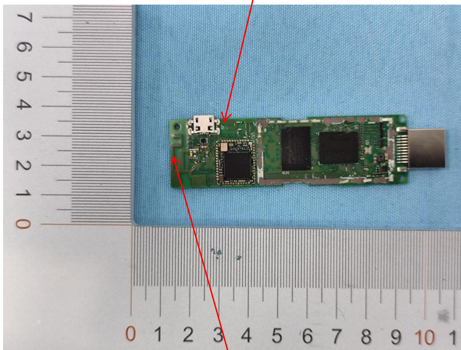
RLAN ANT
