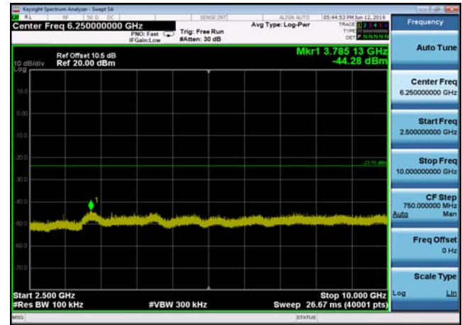
,Plot 4,2500MHz~10000MHz-802.11n(HT20 ) ,2437MHz,Ant1
