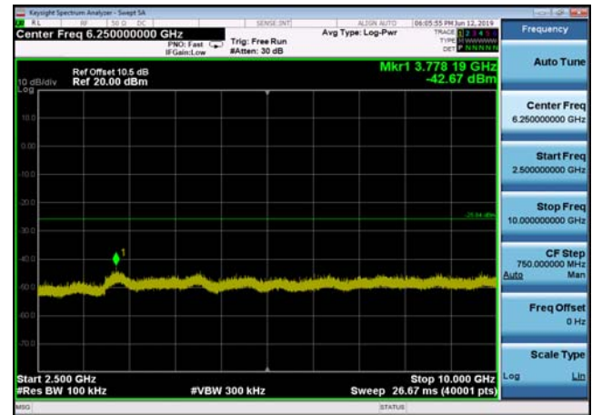
,Plot 4,2500MHz~10000MHz-802.11n(HT20 ) ,2462MHz,Ant1
