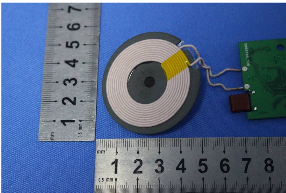
Antenna
