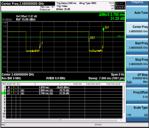
NTNV-DH5-Ant1-2480
