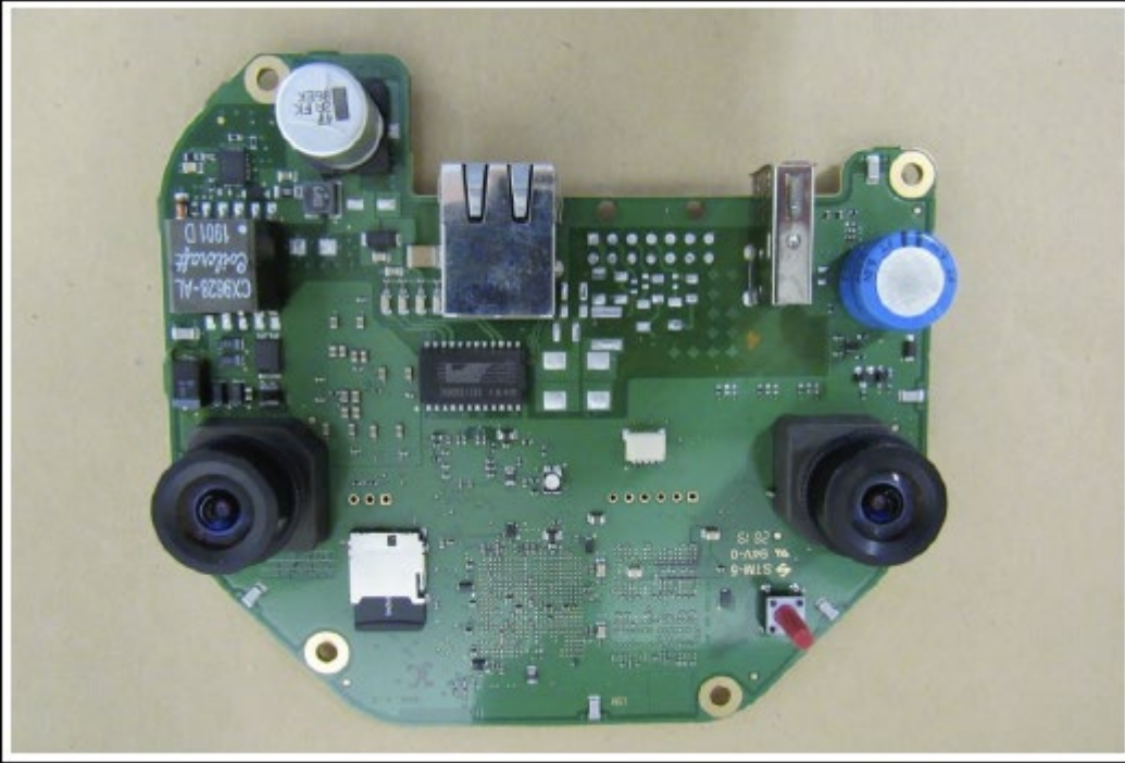
EUT PCB TOP SIDE
