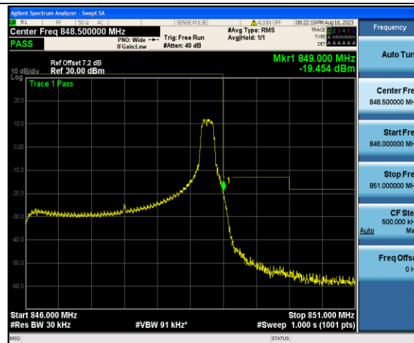
Band5_3MHz_QPSK_20635_1RB#14
