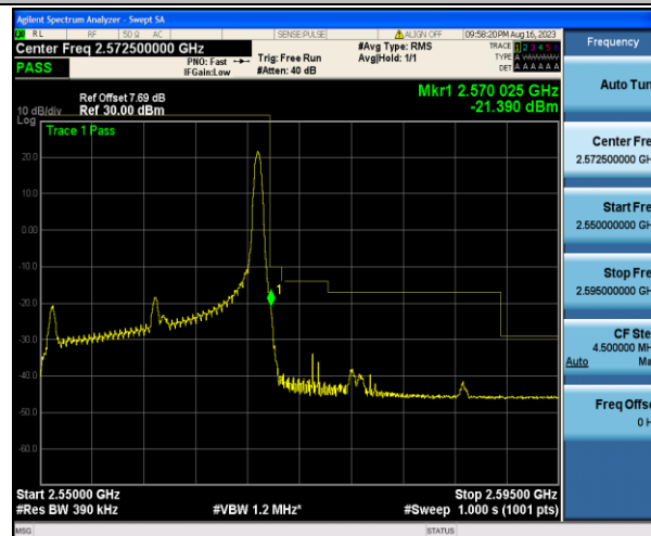
Band7_20MHz_16QAM_21350_1RB#99
