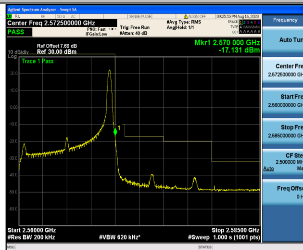
Band7 10MHz QPSK 21400 1RB#49
