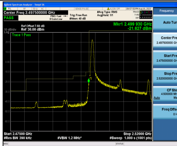
Band7_20MHz_QPSK_20850_1RB#0
