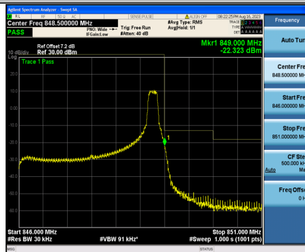
Band5_3MHz_16QAM_20635_1RB#14
