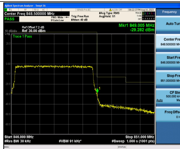
Band5_3MHz_16QAM_20635_15RB#0
