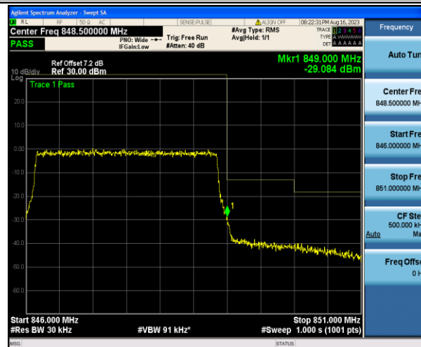
Band5_3MHz_QPSK_20635_15RB#0
