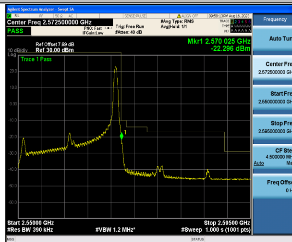
Band7_20MHz_QPSK_21350_1RB#99
