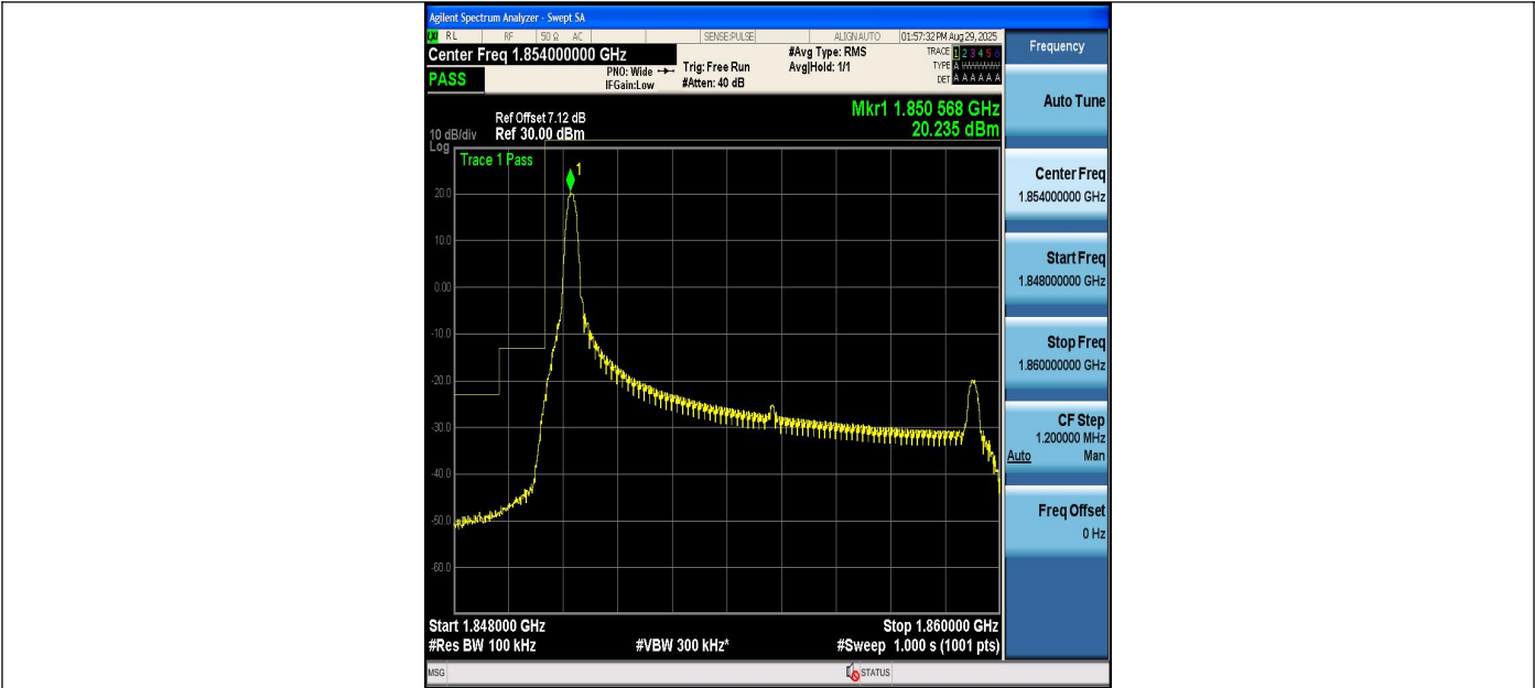
Band2_10MHz_QPSK_18650_1RB#0
