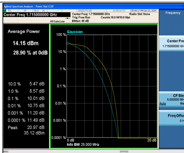
Band4-10MHz-QPSK-20000-50RB#0-PASS
