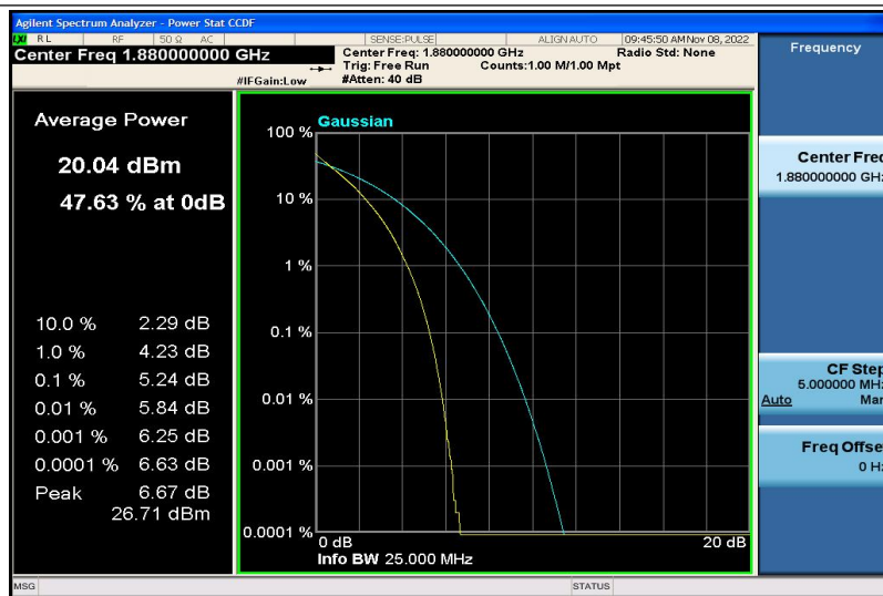
Band2-20MHz-QPSK-18900-100RB#0
