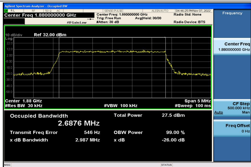
Band2-3MHz-QPSK-18900-15RB#0-2.6876
