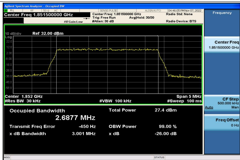
Band2-3MHz-QPSK-18615-15RB#0-2.6877
