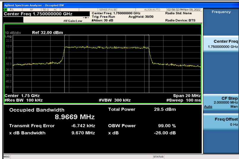
Band4-10MHz-QPSK-20350-50RB#0-8.9669
