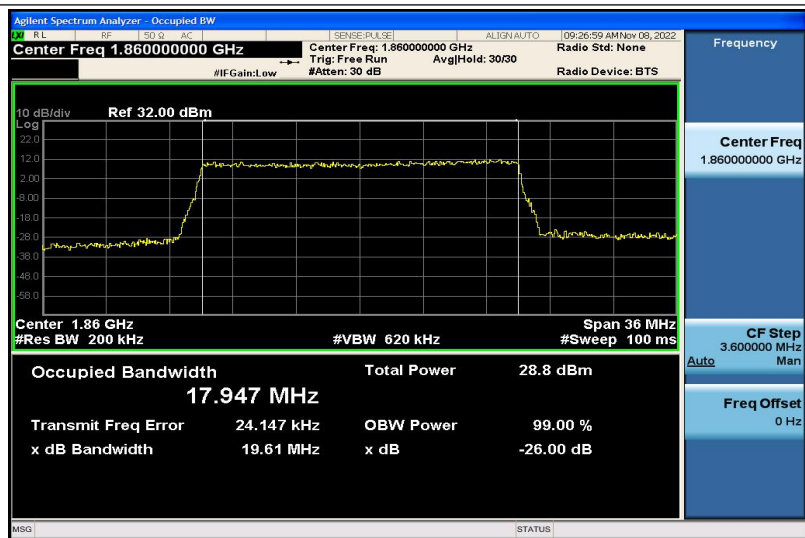
Band2-20MHz-QPSK-18700-100RB#0-17.947
