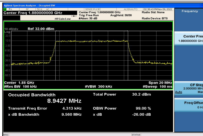
Band2-10MHz-QPSK-18900-50RB#0-8.9427
