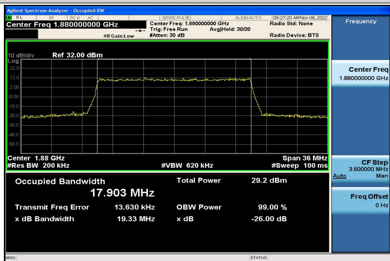
Band2-20MHz-QPSK-18900-100RB#0-17.903
