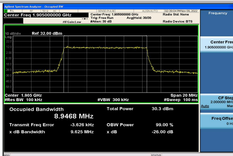
Band2-10MHz-QPSK-19150-50RB#0-8.9468
