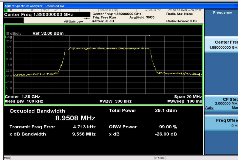
Band2-10MHz-16QAM-18900-50RB#0-8.9508
