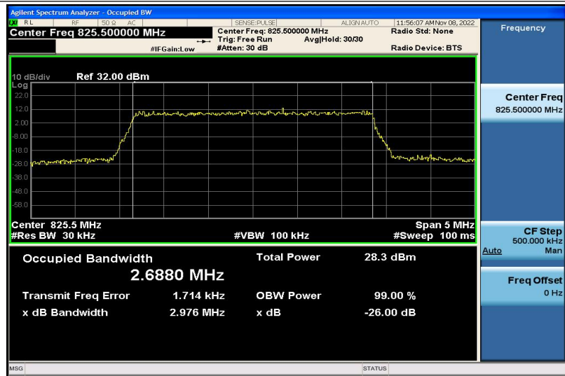
Band5-3MHz-QPSK-20415-15RB#0-2.6880
