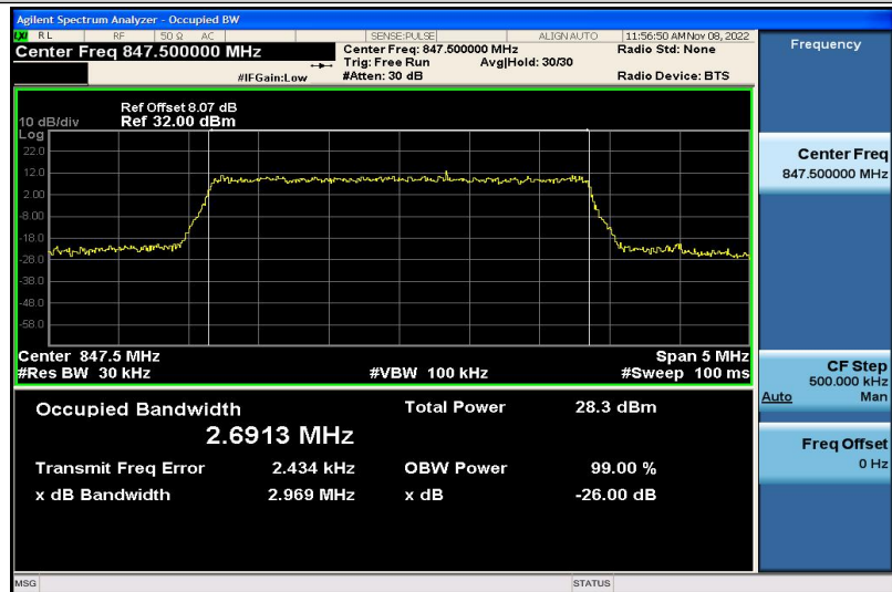
Band5-3MHz-QPSK-20635-15RB#0-2.6913
