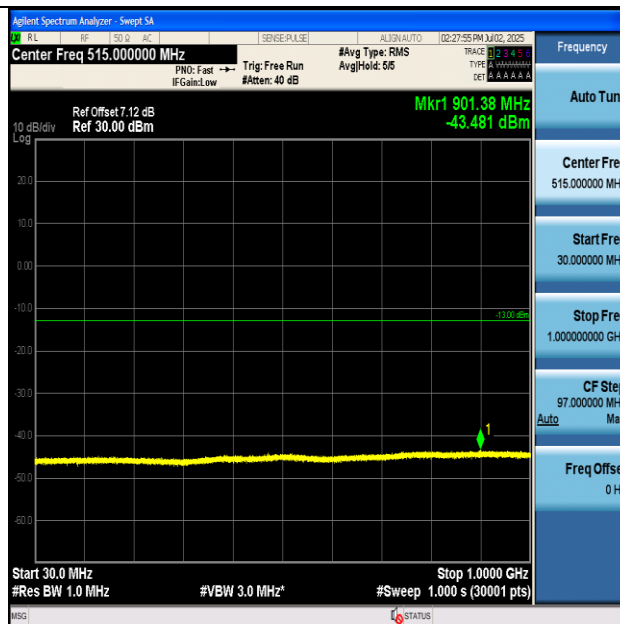
GSM1900-661-0-30~1000MHz-PASS
