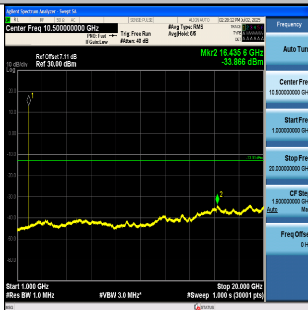
GSM1900-661-0-1000~20000MHz-PASS
