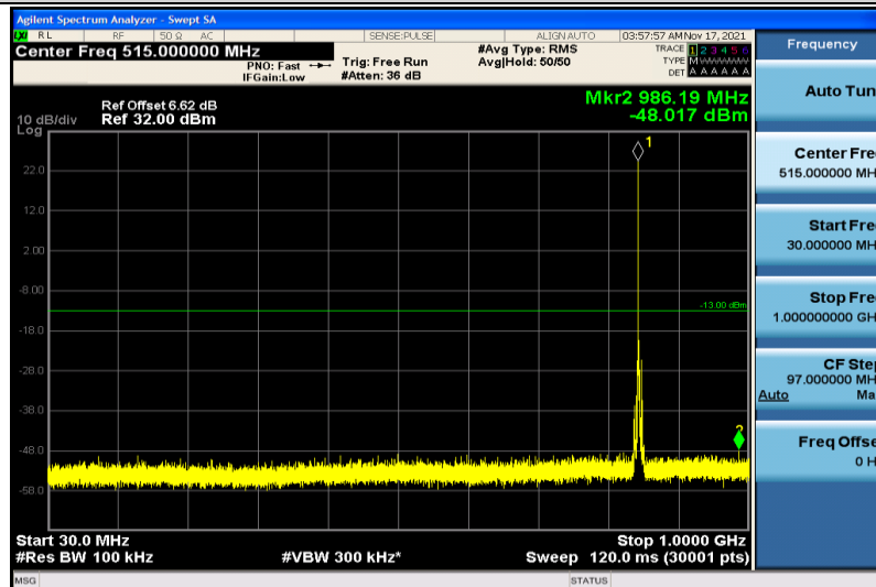
Band5-3MHz-QPSK-20635-1RB#0-30~1000MHz
