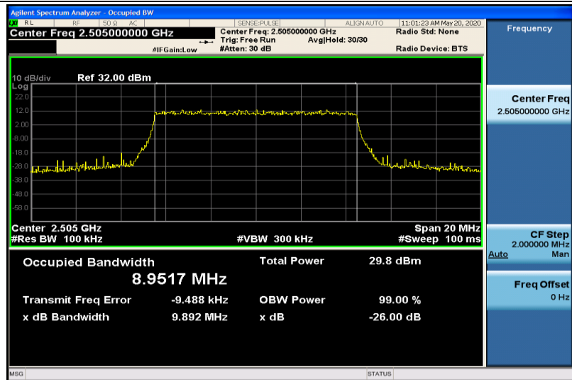
Band7-10MHz-QPSK-20800-50RB#0-8.9517
