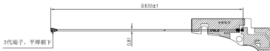
焊接成品图
