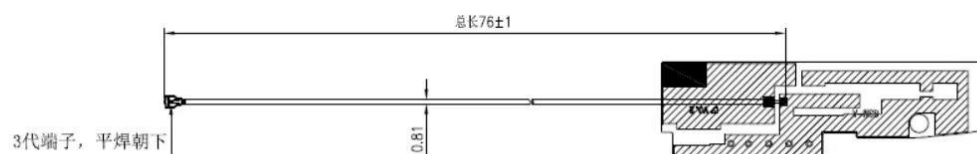
焊接成品图
