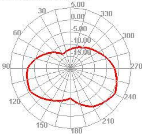
2410.000MHz E2
