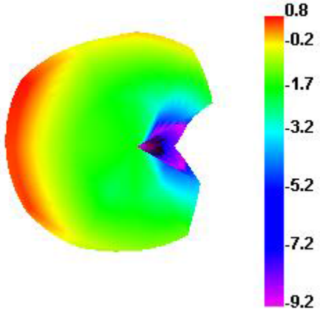
5200.000MHz
