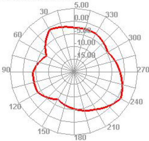
2520.000MHz H
