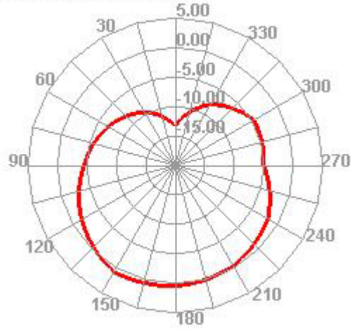
5200.000MHz H
