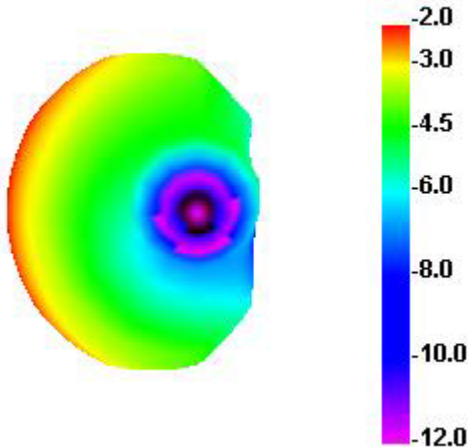
1575.000MHz
