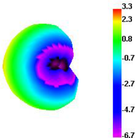
2410.000MHz
