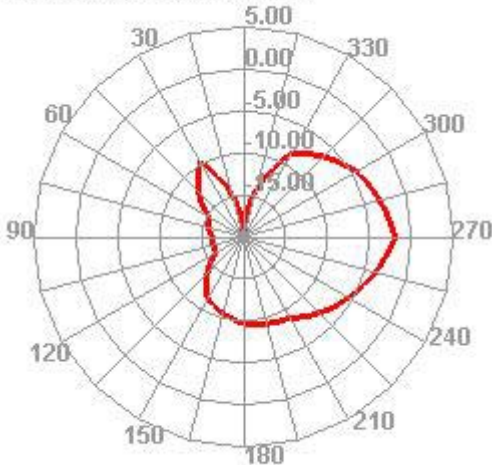
1575.000MHz E1
