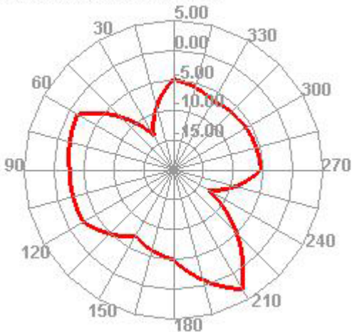
2520.000MHz E1
