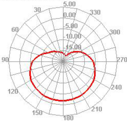
1575.000MHz H
