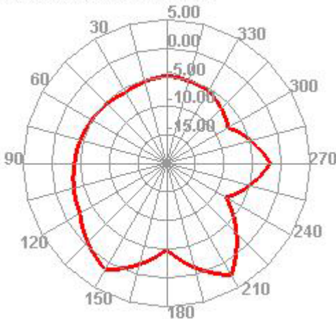
2520.000MHz E2
