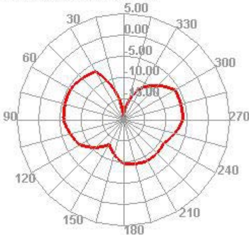
1575.000MHz E2
