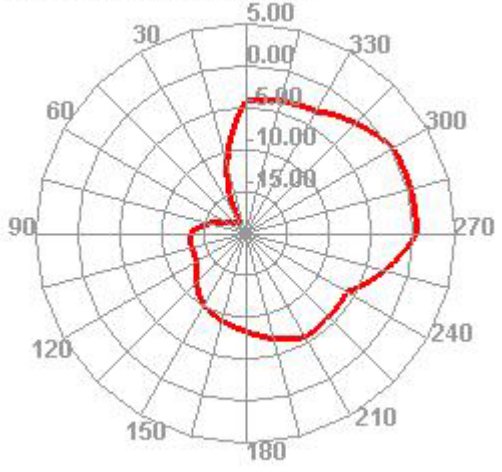
5200.000MHz E1
