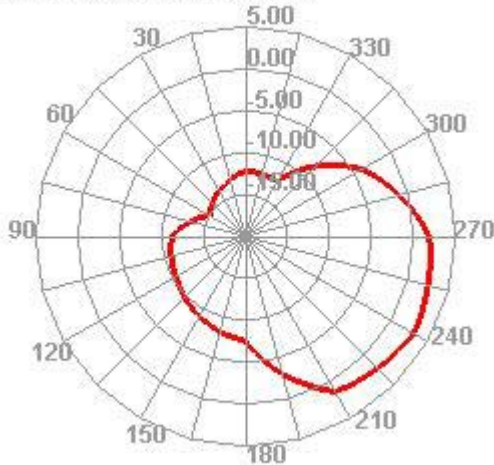
2410.000MHz E1
