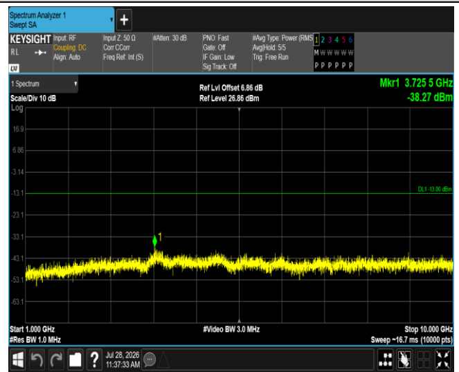
Band12-10MHz-QPSK-23060-1RB#0-Range2:1000~ 10000MHz
