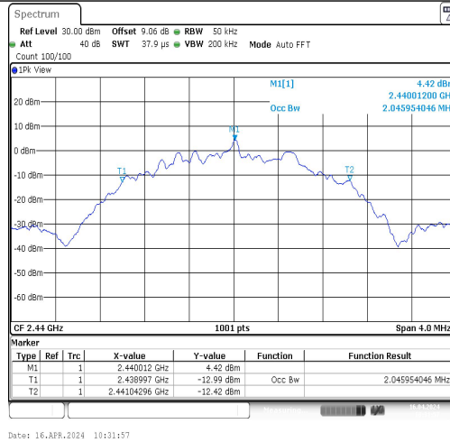
BLE_2M-Ant1-2440
