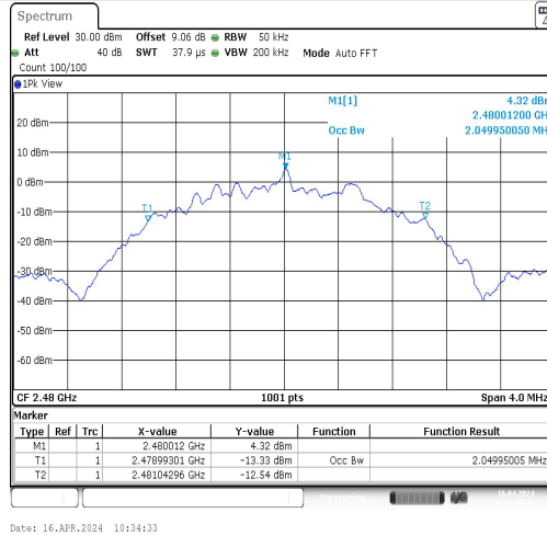
BLE_2M-Ant1-2480
