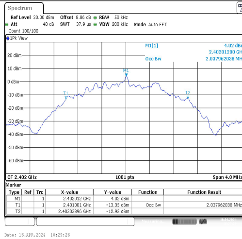
BLE_2M-Ant1-2402
