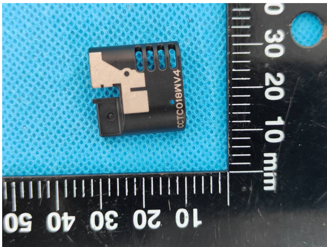
BLE Antenna
