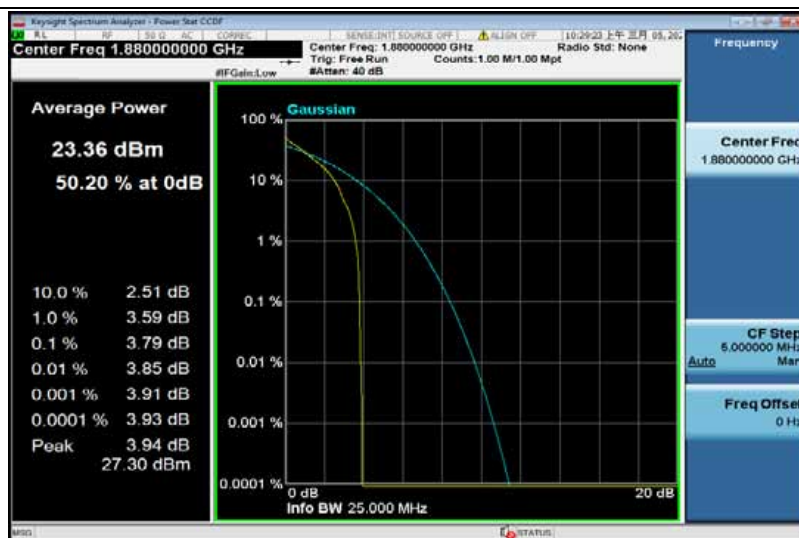
Band2-10MHz-QPSK-18900-50RB#0
