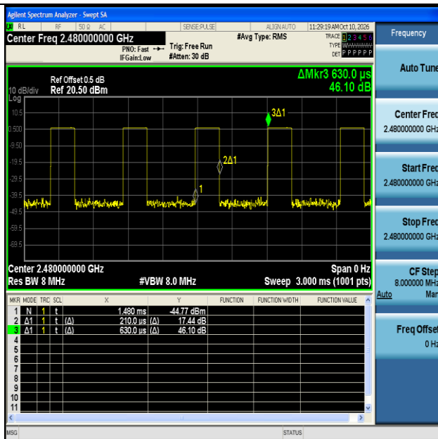
NTNV-SRD-Ant1-2480
