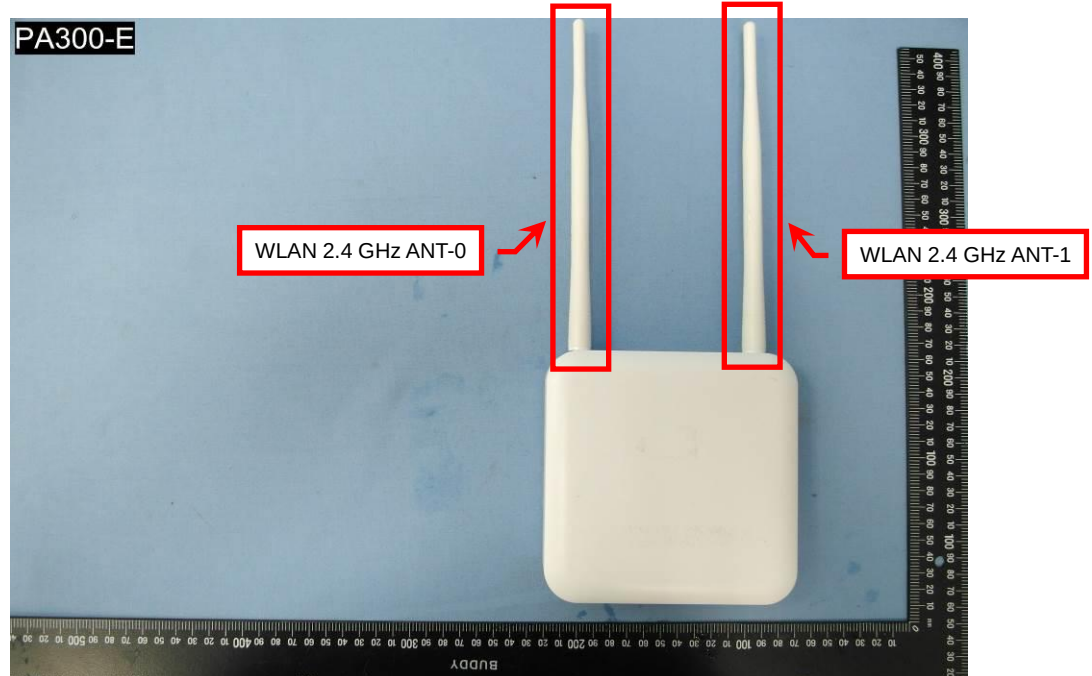
EUT Photo (10)
