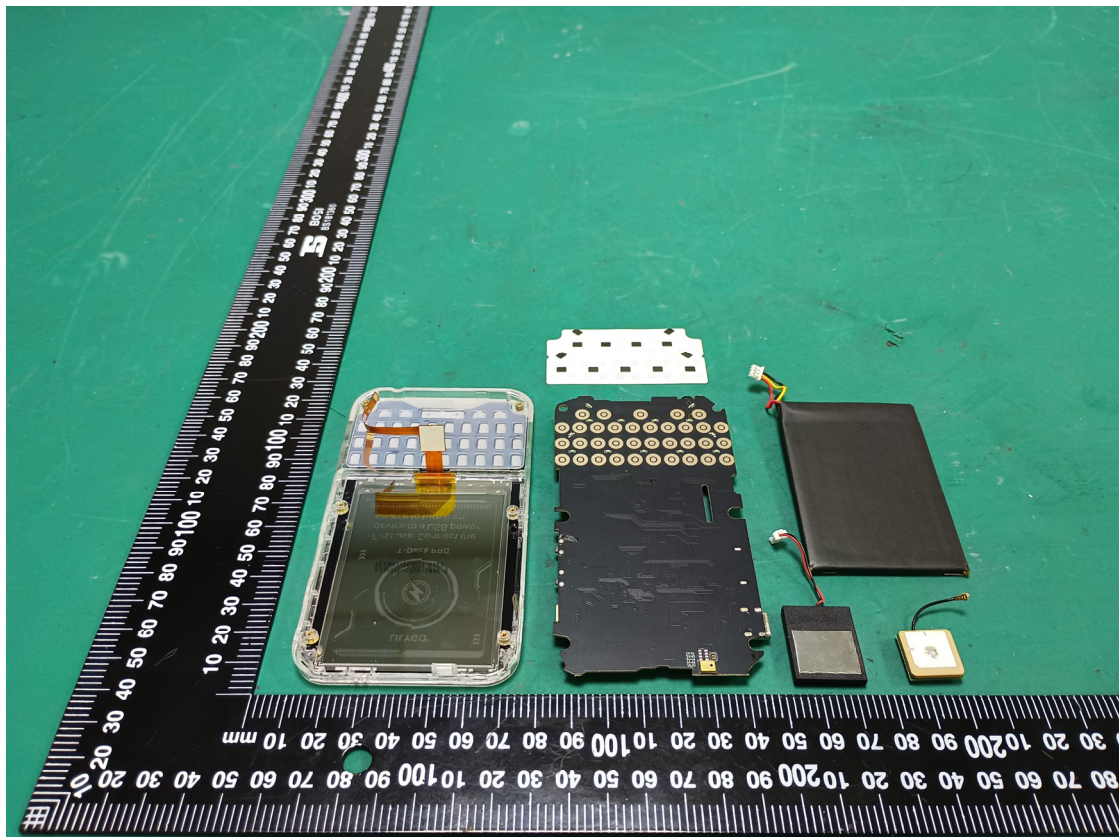
GPS ANT
