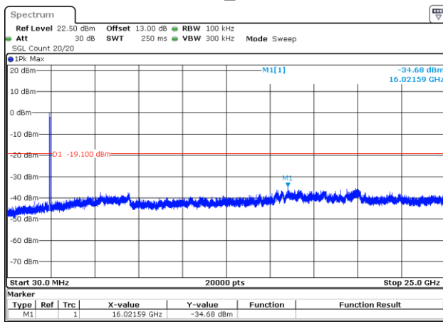
802.11n20_2442MHz
