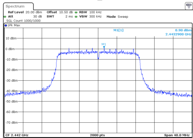
802.11n20_2442MHz
