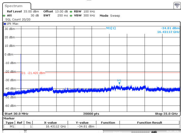
802.11b_2472MHz
