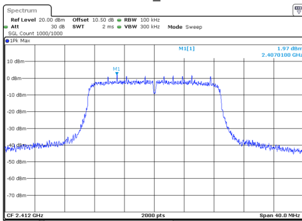
802.11n20_2412MHz
