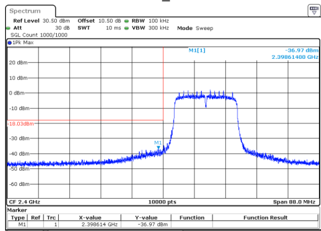
802.11n20_2412MHz
