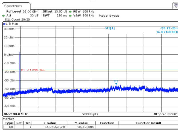
802.11n20_2412MHz
