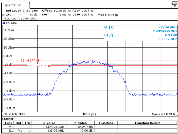
802.11b_2437MHz 9.650MHz
