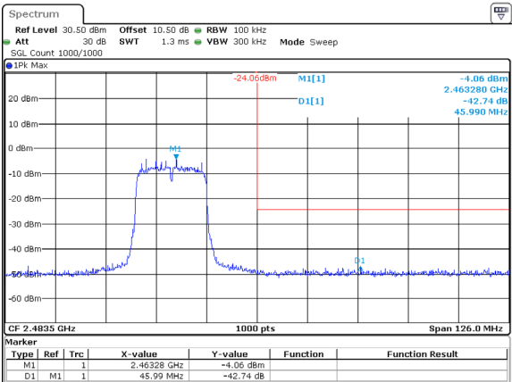
802.11n20_2462MHz
