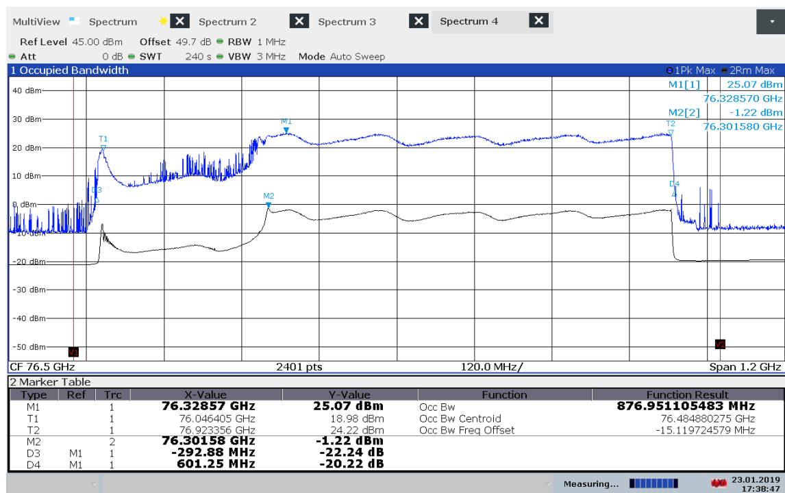
Plot 31: OBW 85 °C
