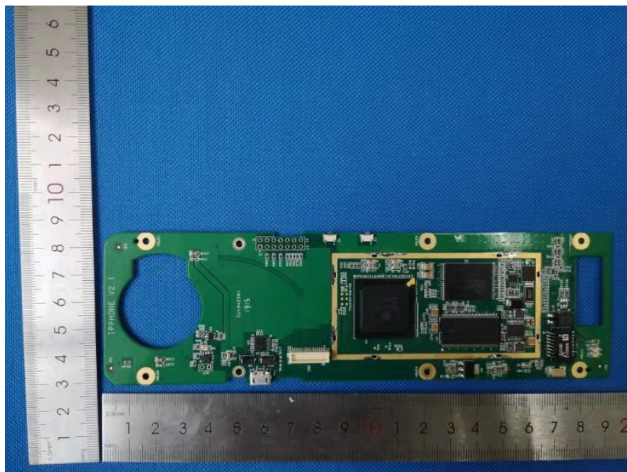
EUT Photo 41
