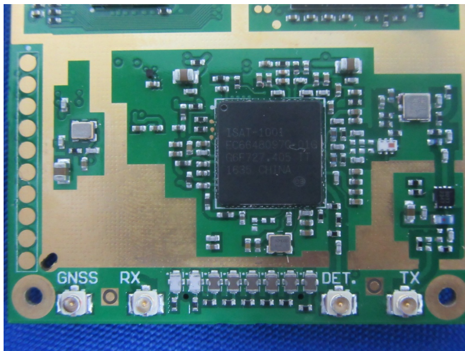
EUT Photo 31
