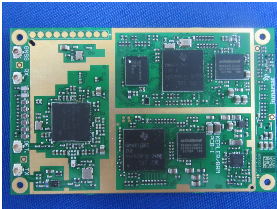
EUT Photo 30
