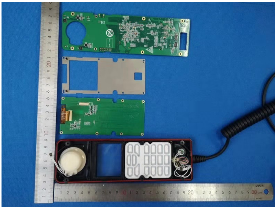
EUT Photo 39
