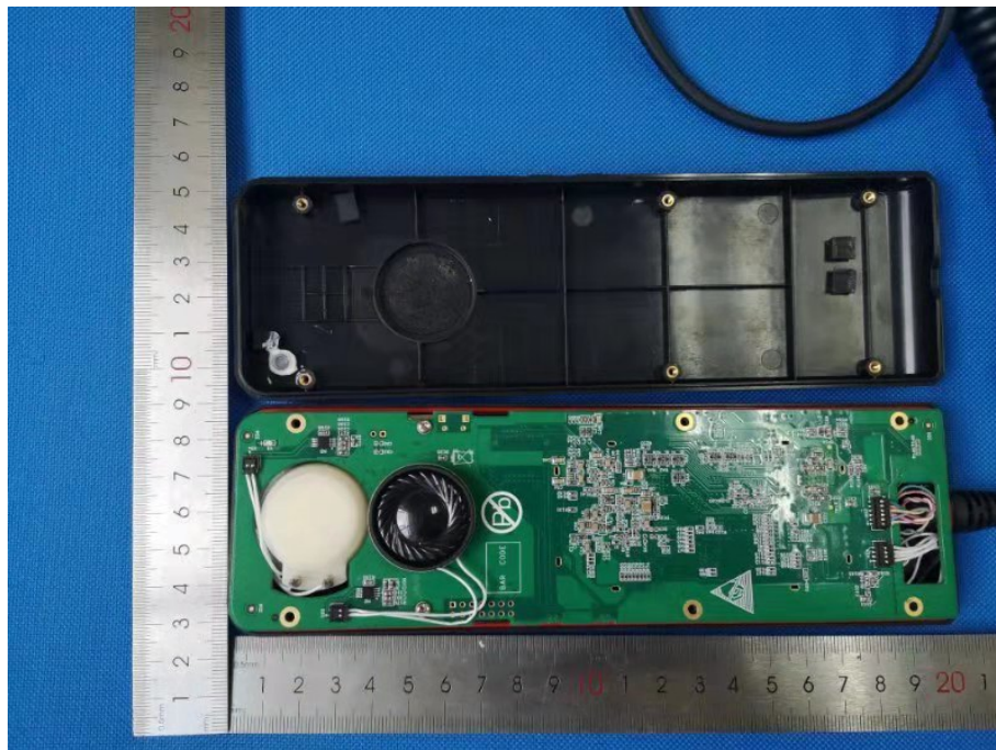
EUT Photo 40
