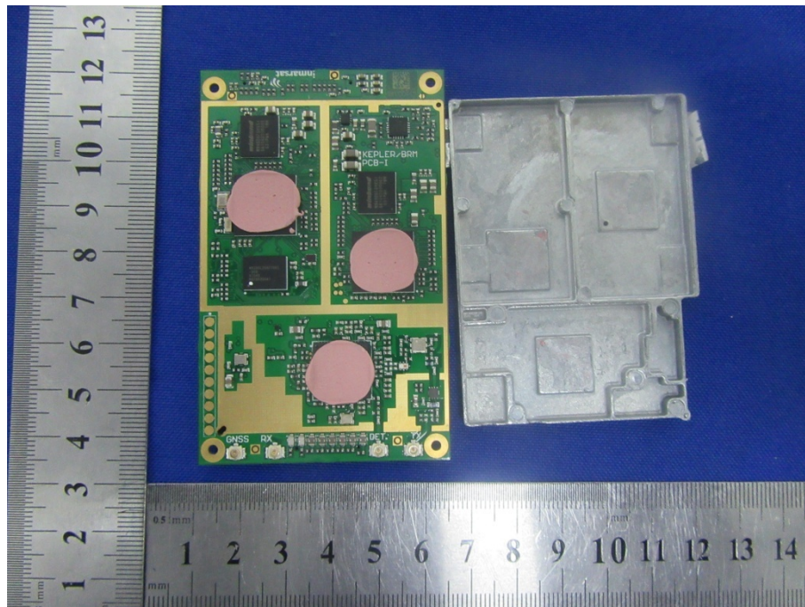
EUT Photo 28
