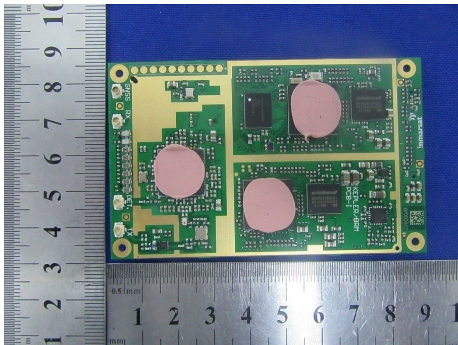
EUT Photo 29
