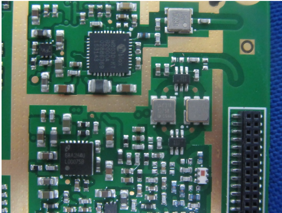
EUT Photo 24
