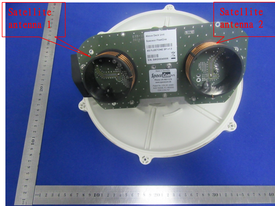
EUT Photo 36
