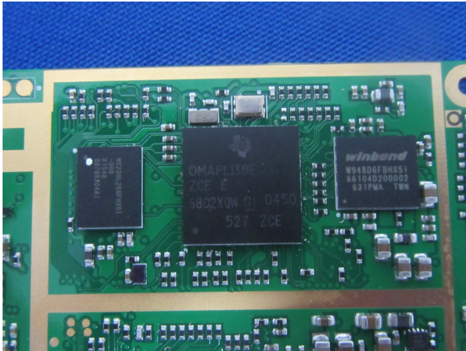
EUT Photo 32
