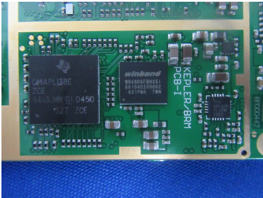
EUT Photo 33
