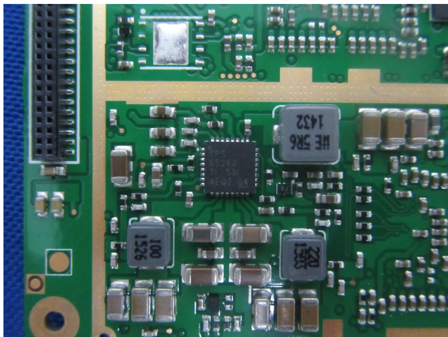
EUT Photo 27
