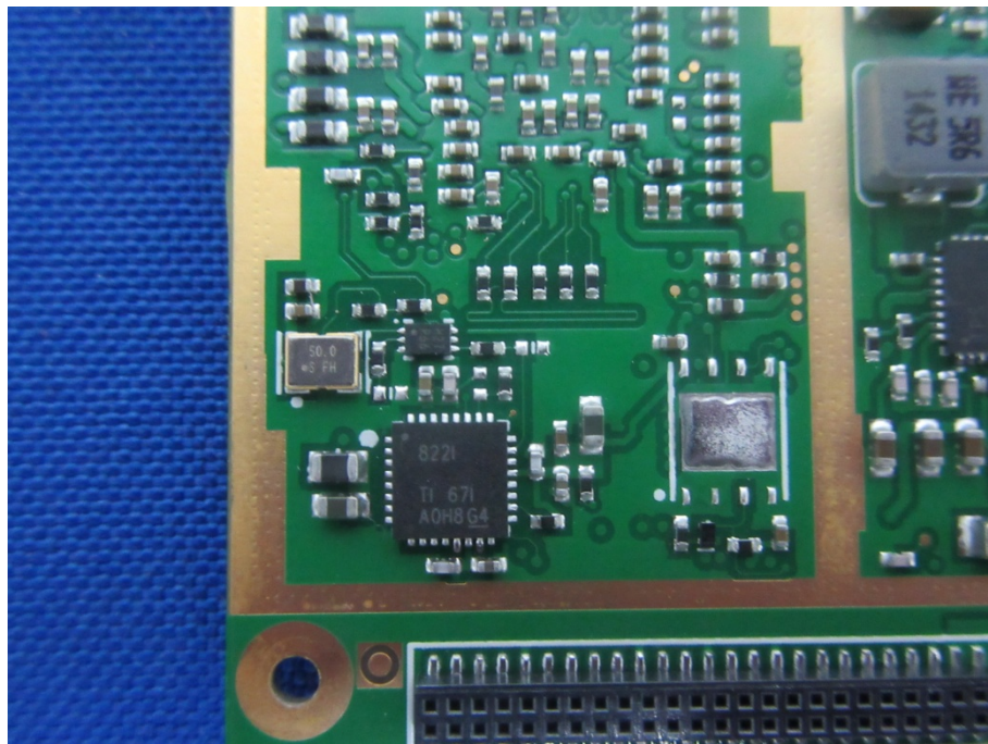
EUT Photo 26
