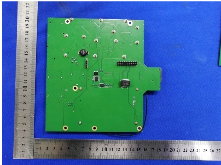
EUT Photo 15
