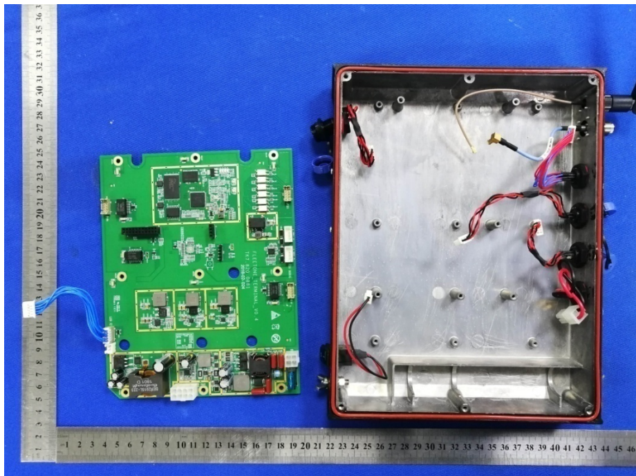
EUT Photo 11
