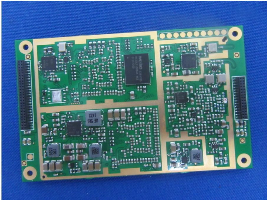
EUT Photo 22
