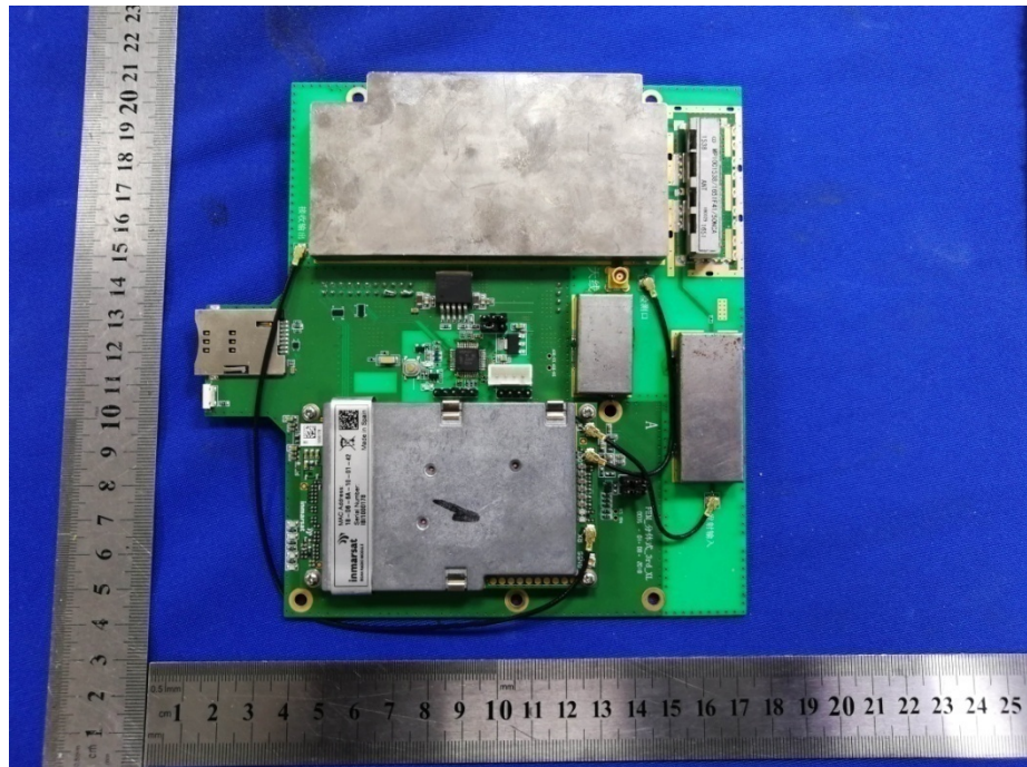
EUT Photo 14
