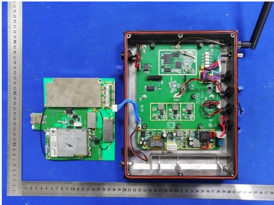
EUT Photo 10
