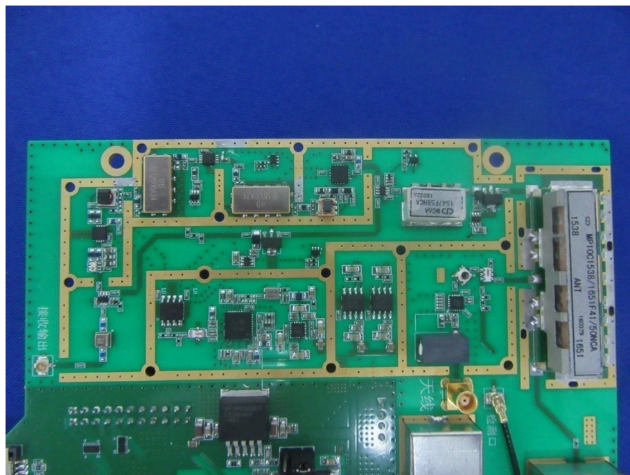
EUT Photo 17
