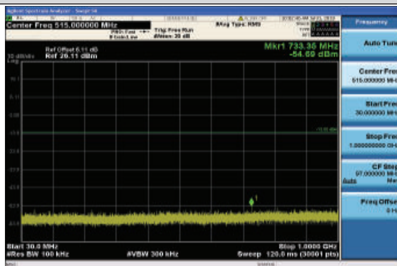
Band4-1.4MHz-QPSK-20393-1RB#0-30~1000MHz
