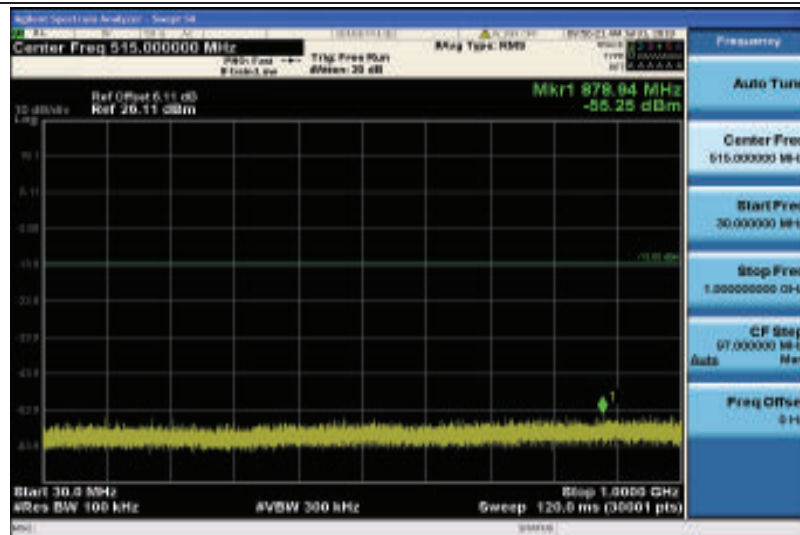
Band2-20MHz-QPSK-18900-1RB#0-30~1000MHz
