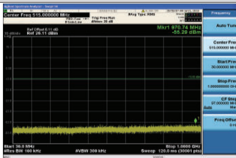
Band2-20MHz-16QAM-19100-1RB#0-30~1000MHz
