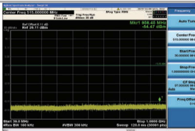
Band2-20MHz-QPSK-19100-1RB#0-30~1000MHz
