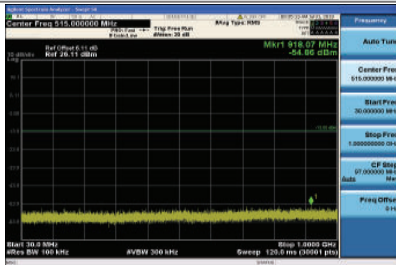
Band2-5MHz-QPSK-18625-1RB#0-30~1000MHz
