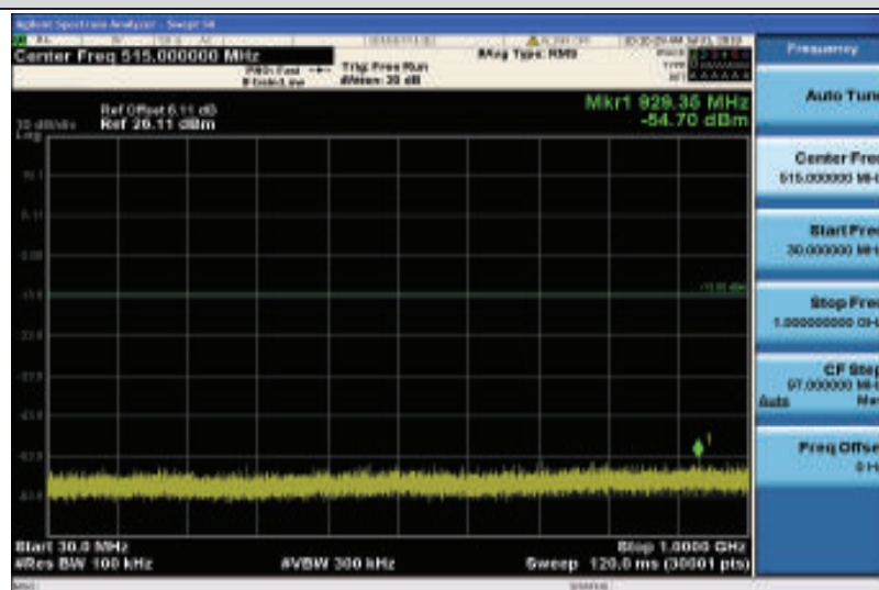
Band4-5MHz-QPSK-20375-1RB#0-30~1000MHz
