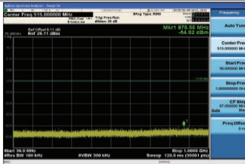
Band2-20MHz-16QAM-18900-1RB#0-30~1000MHz
