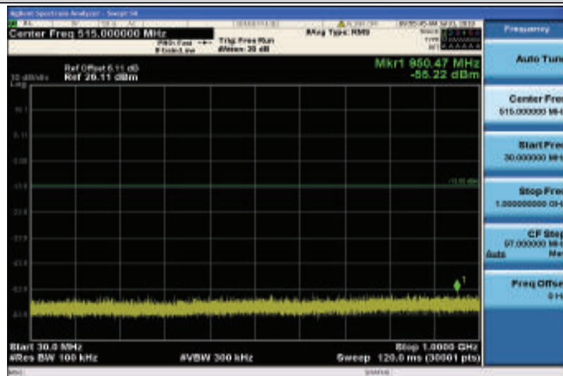
Band2-20MHz-16QAM-18700-1RB#0-30~1000MHz
