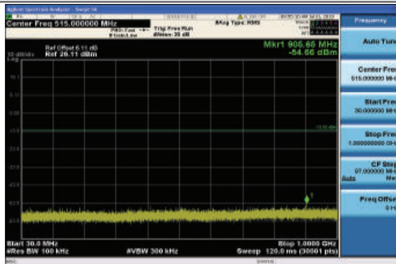
Band2-20MHz-QPSK-18700-1RB#0-30~1000MHz
