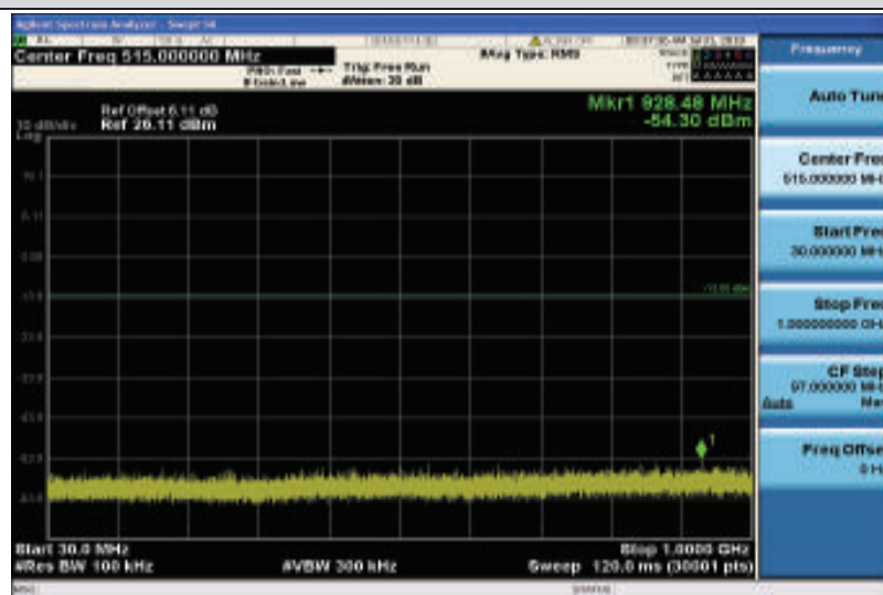
Band2-5MHz-QPSK-19175-1RB#0-30~1000MHz
