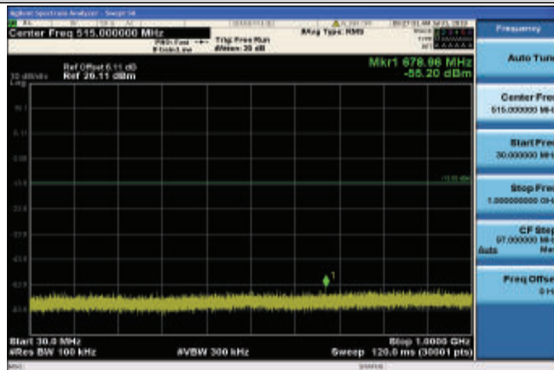
Band2-3MHz-QPSK-18615-1RB#0-30~1000MHz
