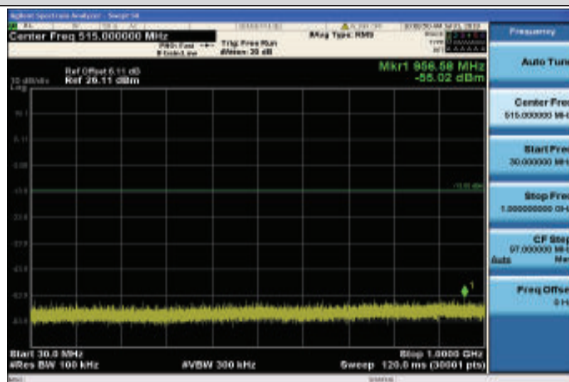
Band4-3MHz-QPSK-20385-1RB#0-30~1000MHz
