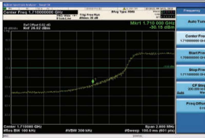
Band4-10MHz-QPSK-20000-50RB#0
