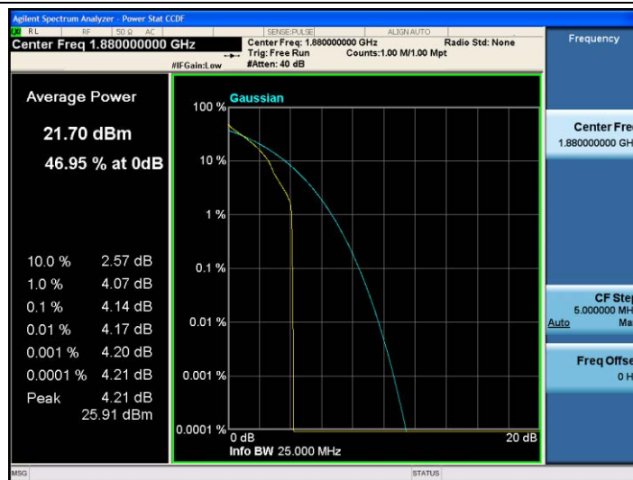
Band2-20MHz-QPSK-18900-1RB#0
