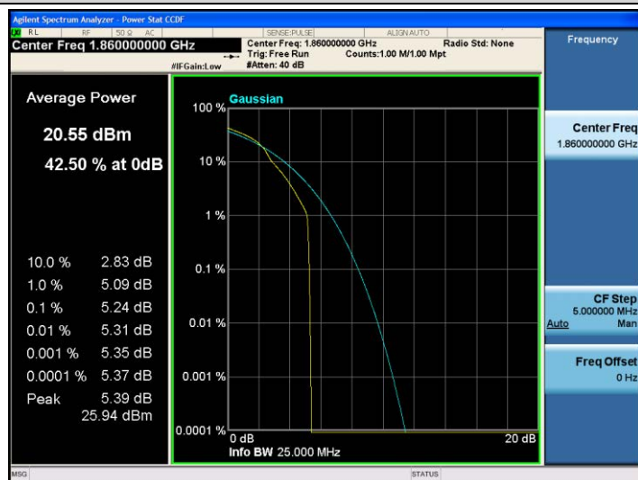
Band2-20MHz-16QAM-18700-1RB#0
