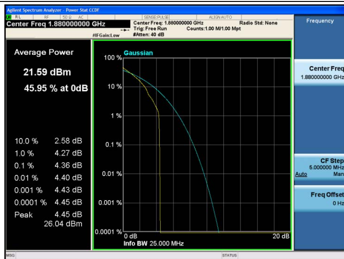
Band2-10MHz-QPSK-18900-1RB#0
