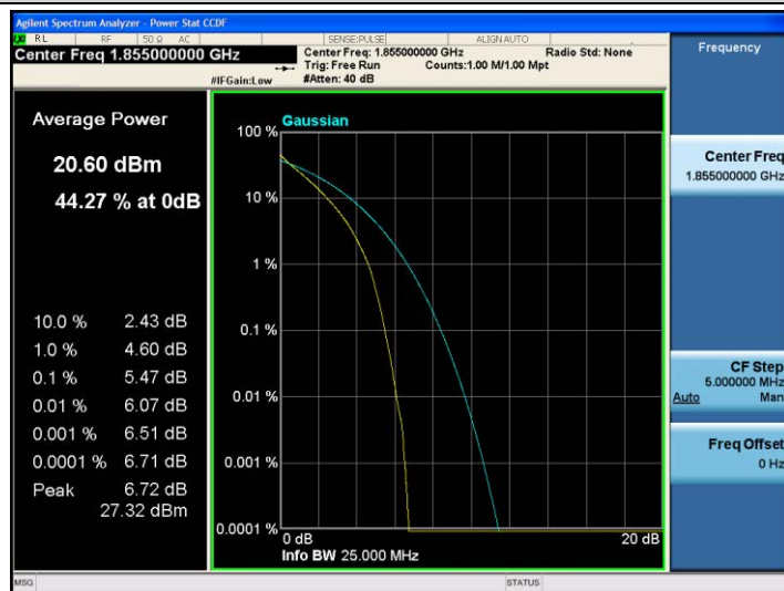
Band2-10MHz-QPSK-18650-50RB#0
