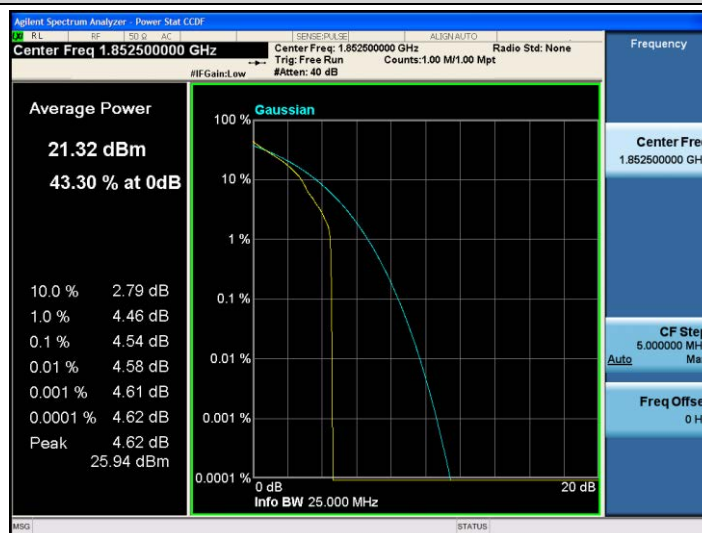
Band2-5MHz-QPSK-18625-1RB#0
