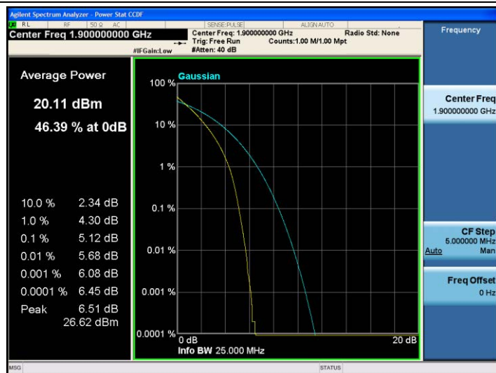
Band2-20MHz-QPSK-19100-100RB#0
