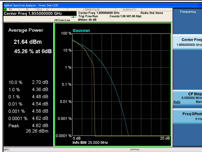
Band2-10MHz-QPSK-18650-1RB#0
