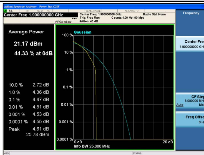
Band2-20MHz-QPSK-19100-1RB#0
