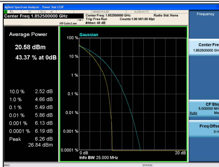
Band2-5MHz-QPSK-18625-25RB#0
