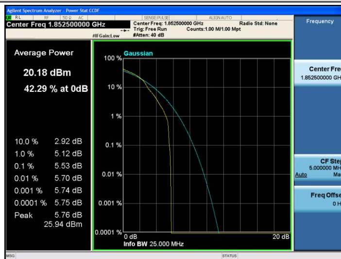
Band2-5MHz-16QAM-18625-1RB#0
