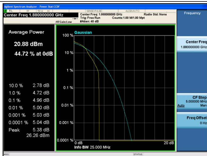
Band2-20MHz-16QAM-18900-1RB#0
