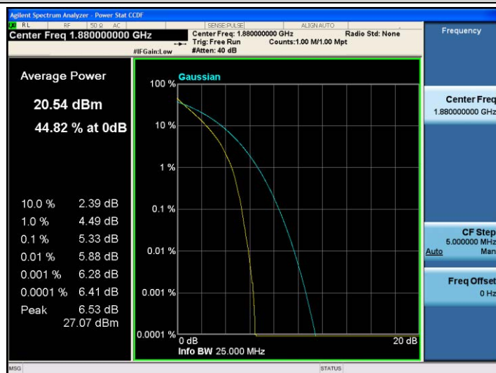
Band2-10MHz-QPSK-18900-50RB#0
