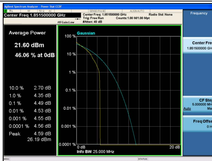
Band2-3MHz-QPSK-18615-1RB#0
