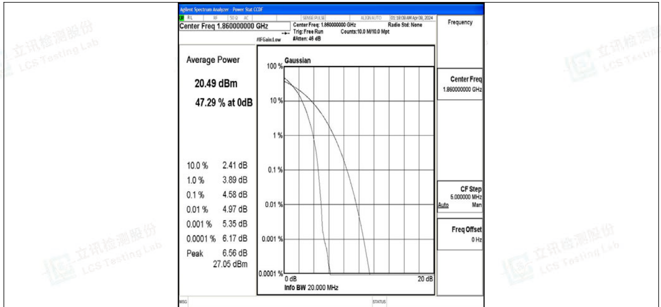
Band2-20MHz-QPSK-18700-1RB#0-PASS
