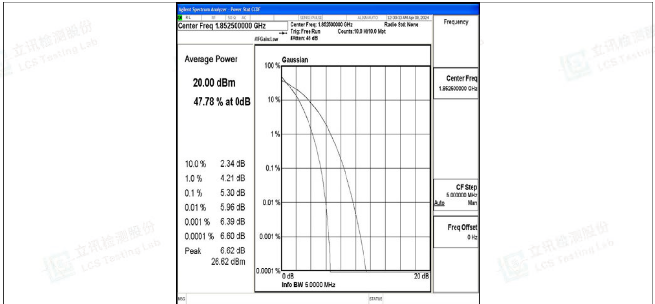
Band2-5MHz-QPSK-18625-25RB#0-PASS
