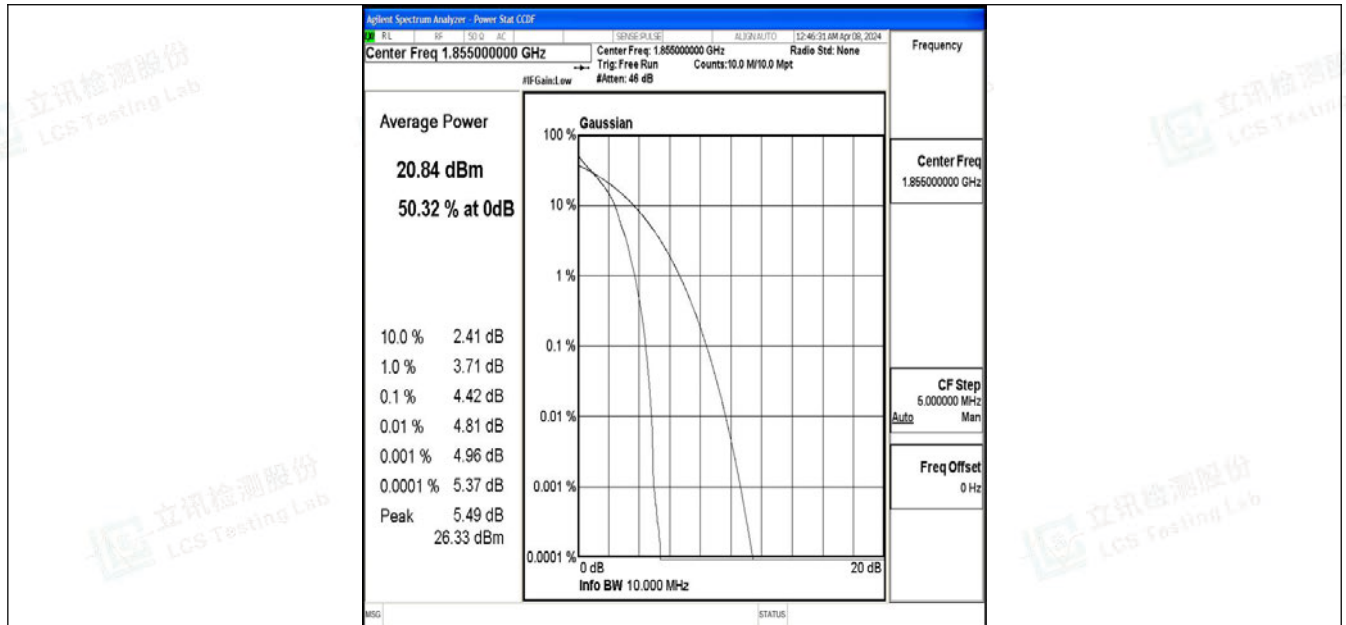
Band2-10MHz-QPSK-18650-1RB#0-PASS
