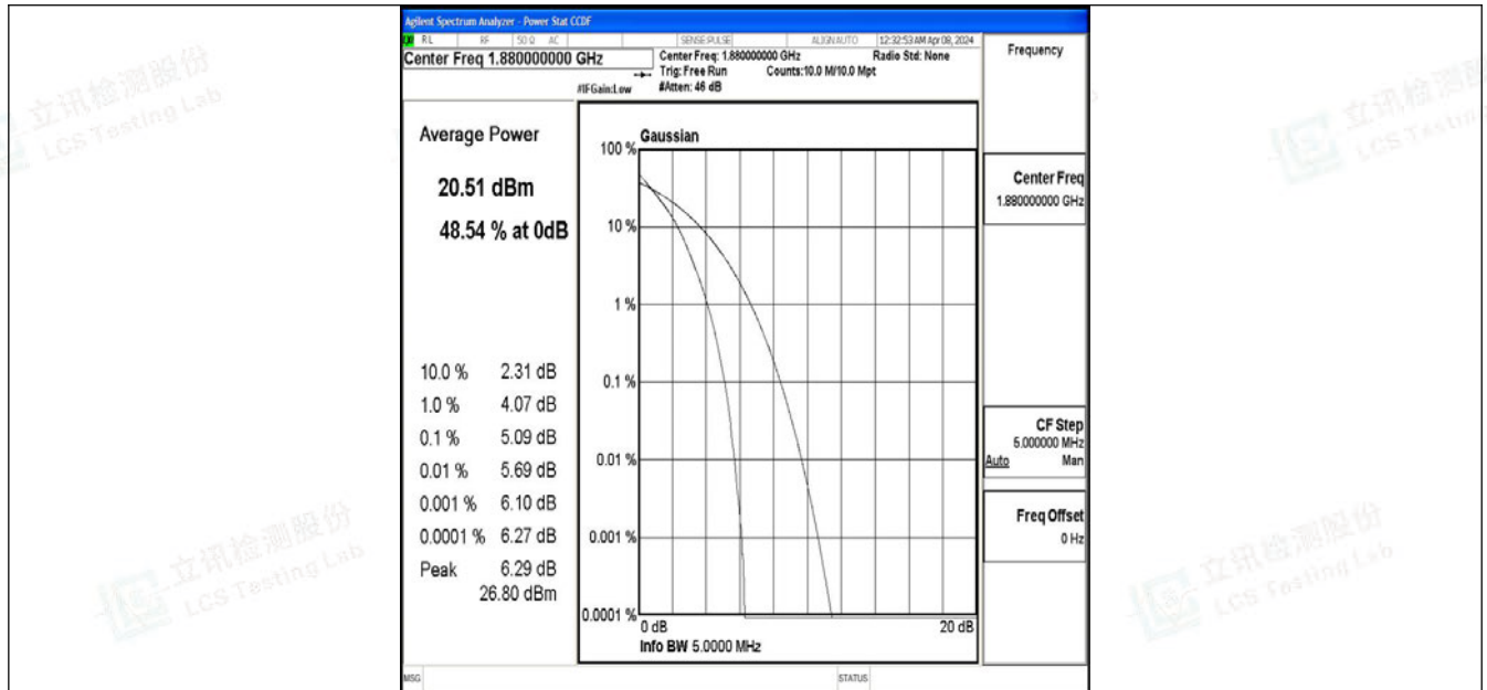
Band2-5MHz-QPSK-18900-25RB#0-PASS
