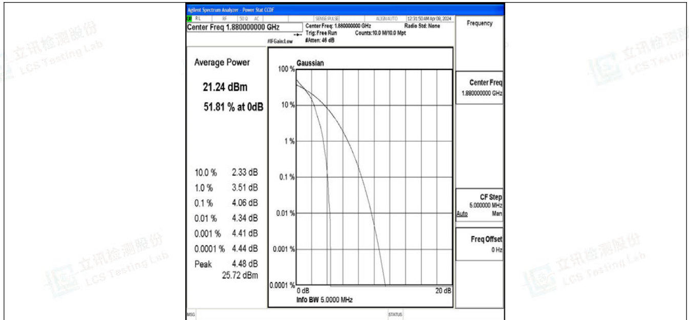
Band2-5MHz-QPSK-18900-1RB#0-PASS
