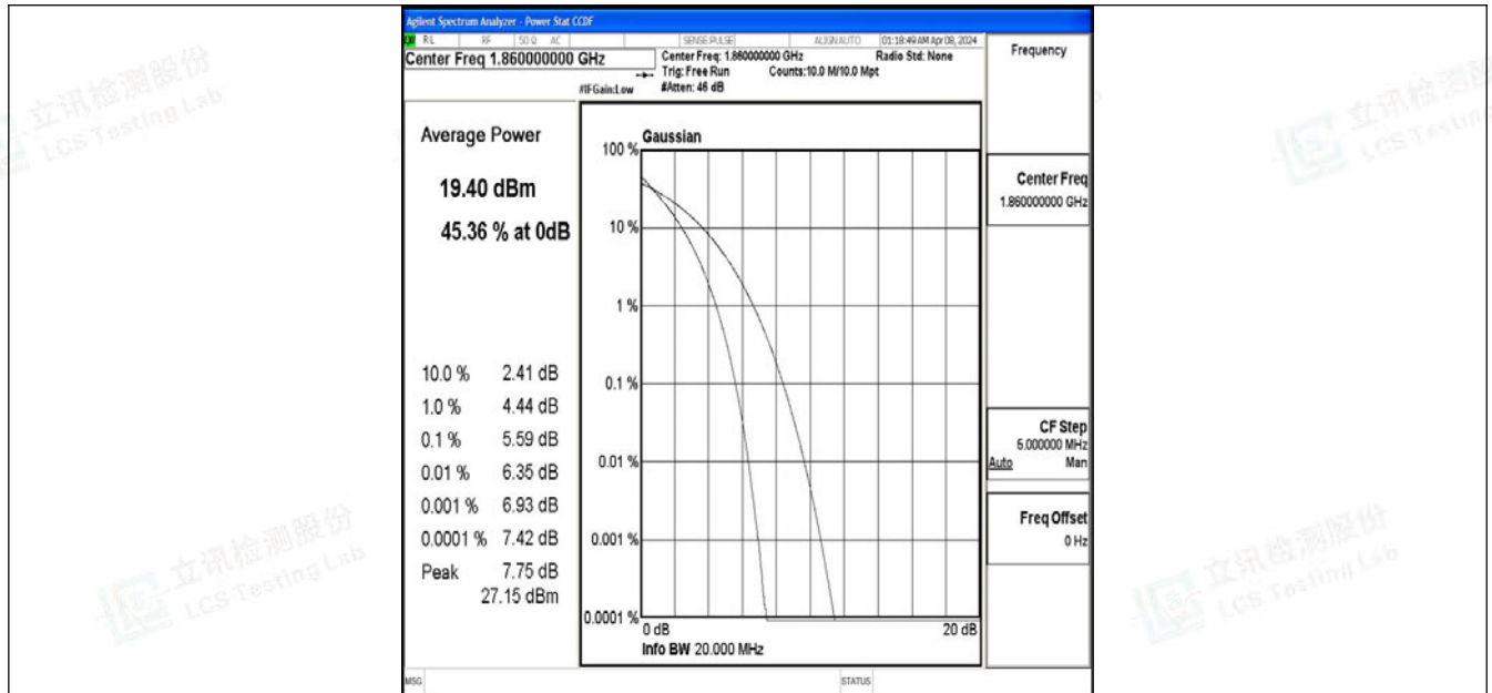
Band2-20MHz-QPSK-18700-100RB#0-PASS
