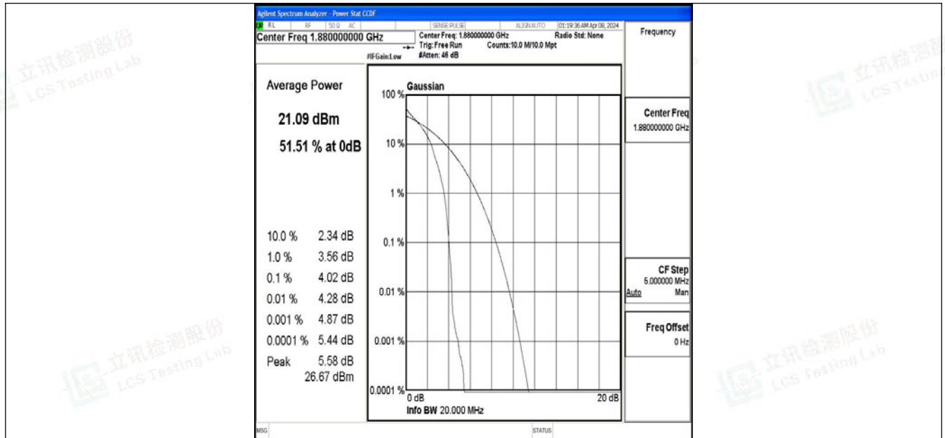
Band2-20MHz-QPSK-18900-1RB#0-PASS
