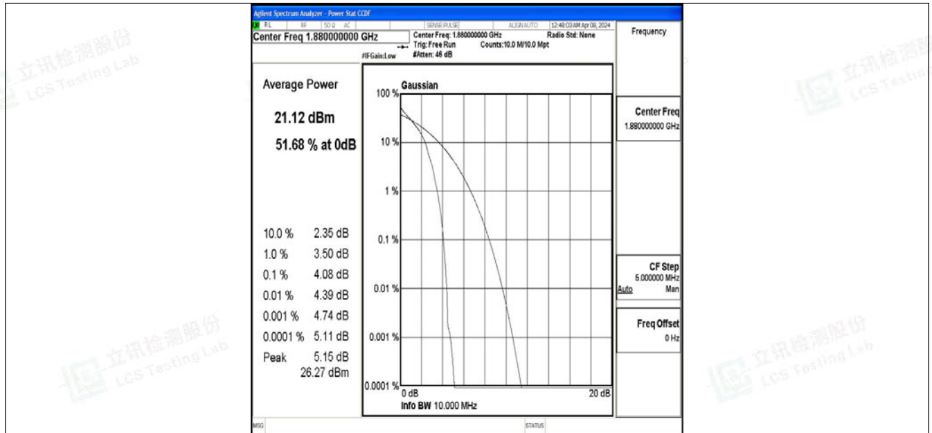
Band2-10MHz-QPSK-18900-1RB#0-PASS
