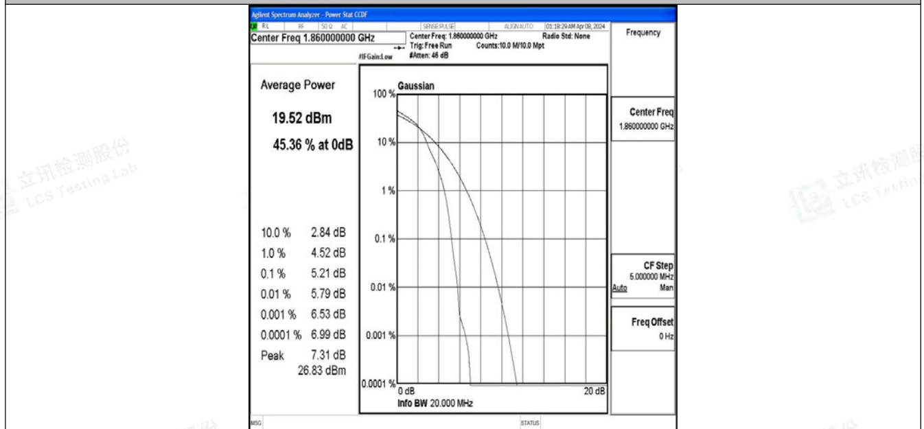
Band2-20MHz-64QAM-18700-1RB#0-PASS
