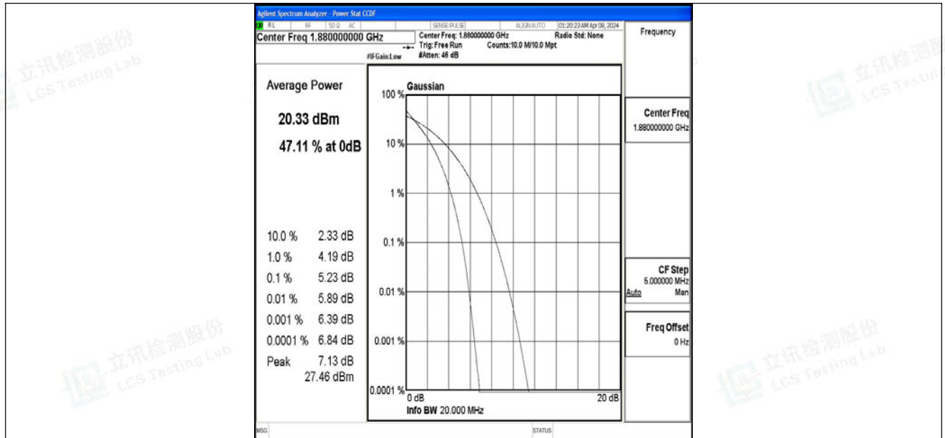
Band2-20MHz-QPSK-18900-100RB#0-PASS
