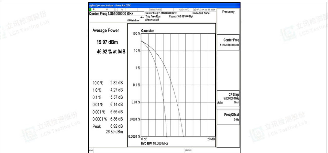
Band2-10MHz-QPSK-18650-50RB#0-PASS
