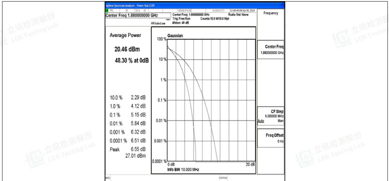
Band2-10MHz-QPSK-18900-50RB#0-PASS
