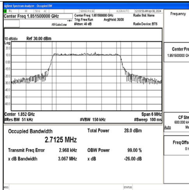
Band2-3MHz-QPSK-18615-15RB#0-PASS
