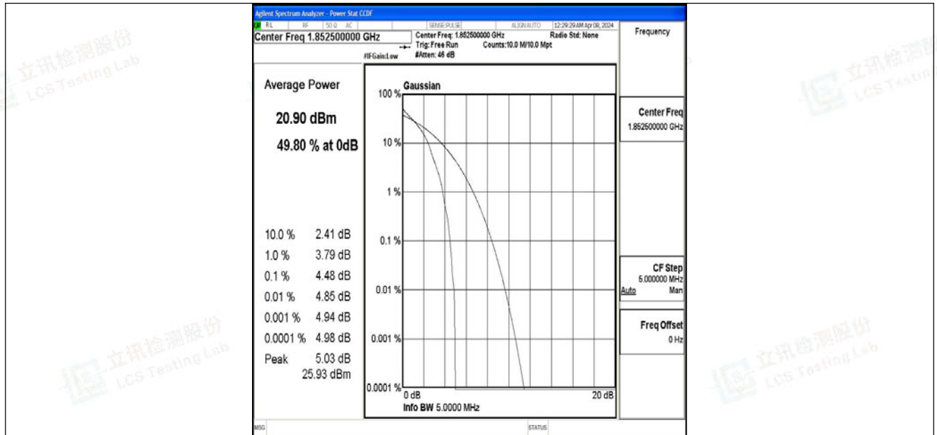
Band2-5MHz-QPSK-18625-1RB#0-PASS
