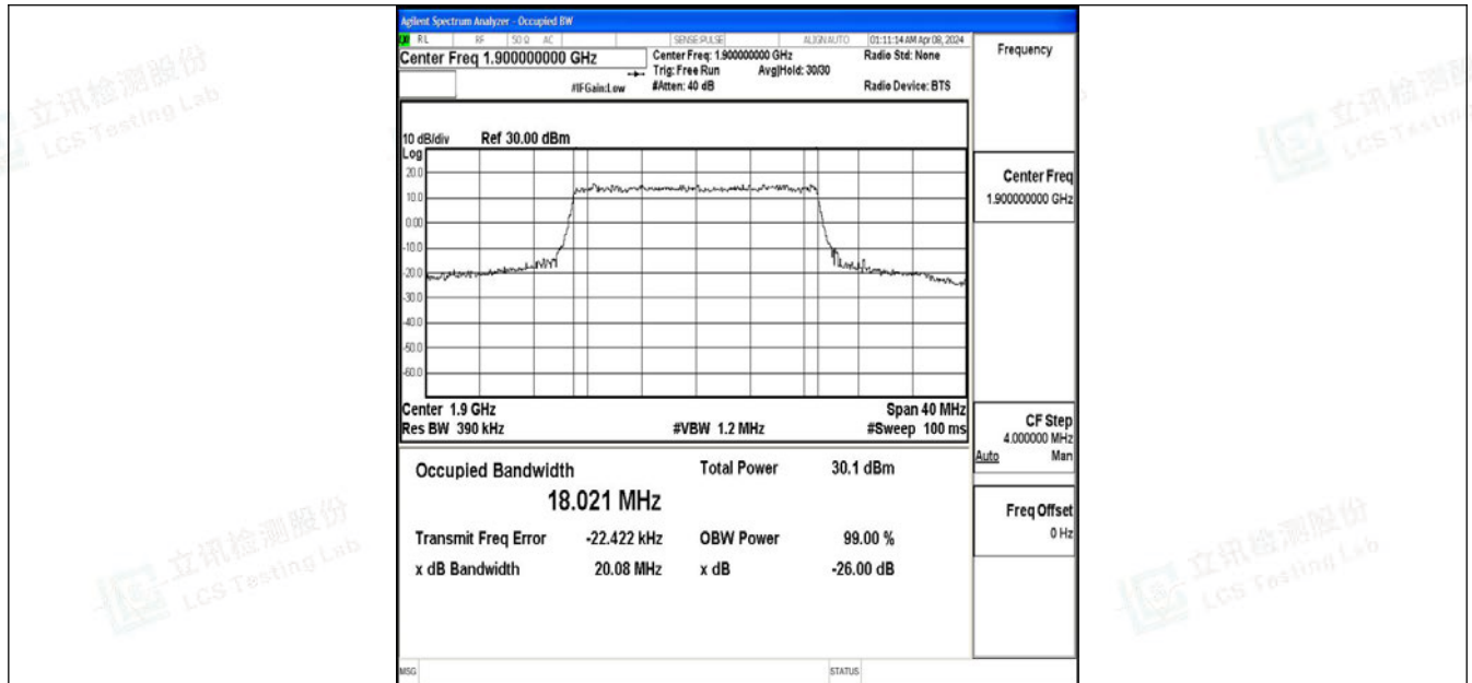
Band2-20MHz-QPSK-19100-100RB#0-PASS
