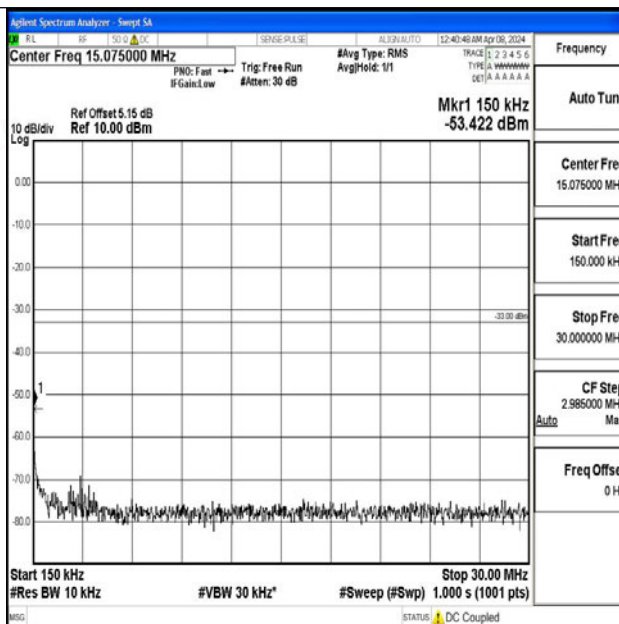
Band2 10MHz QPSK 18650 1RB#0 0.15~30 0.15~30
