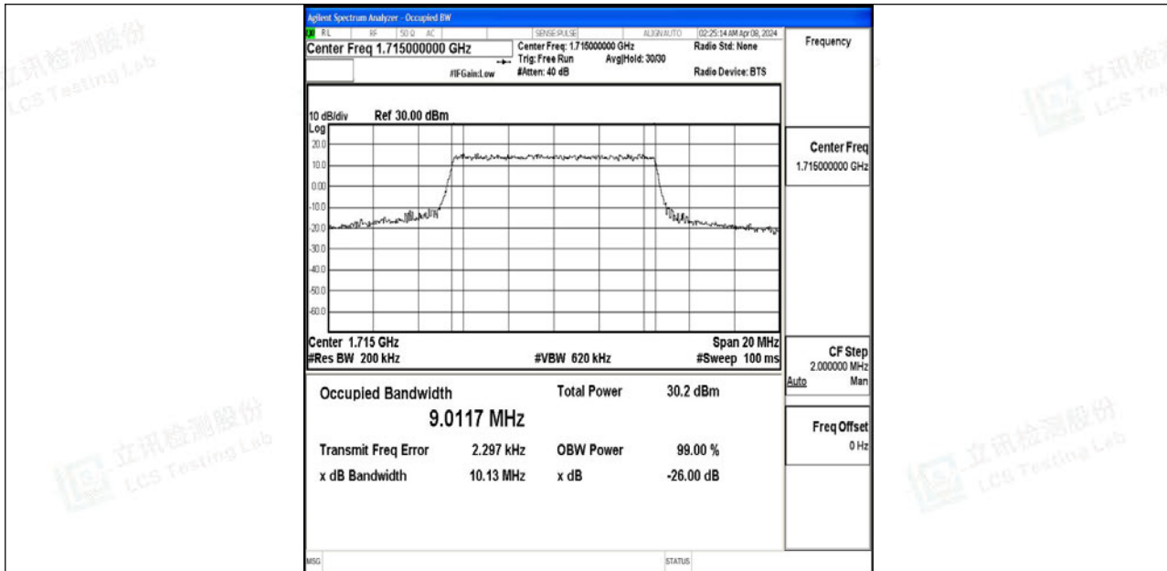
Band4-10MHz-QPSK-20000-50RB#0-PASS
