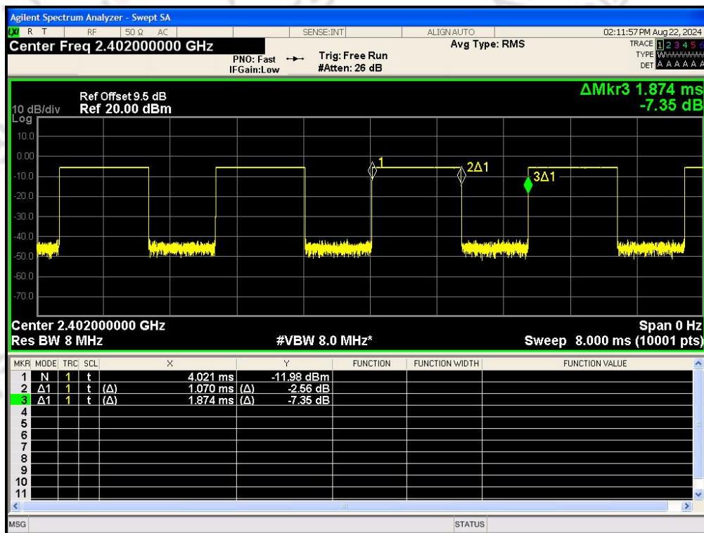
BLE 2M_Channel 0
