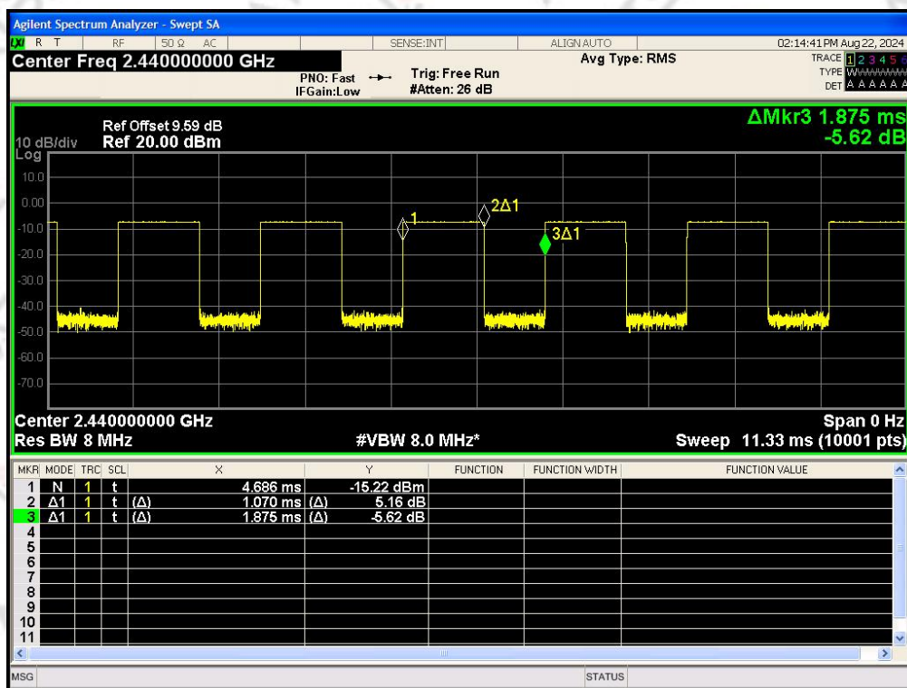
BLE 2M_Channel 19
