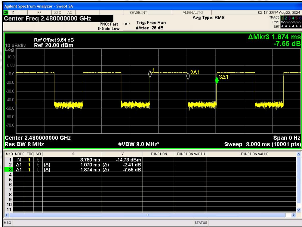
BLE 2M_Channel 39
