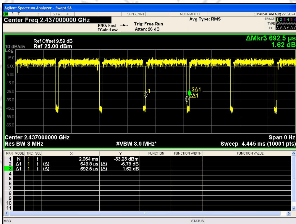
IEEE 802.11n_40MHz_Channel 6
