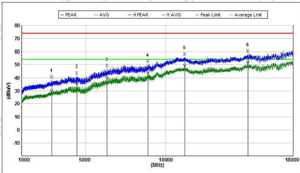
DH5 2402 Horizontal
