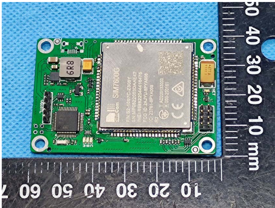
WWAN Module FCC ID: 2AJYU-8PYA008
