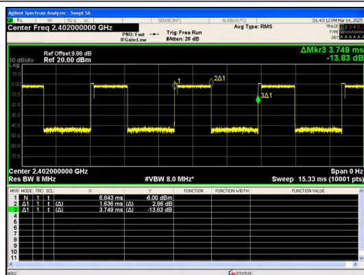
\pi/4 DQPSK(2-DH3)_Channel 0
