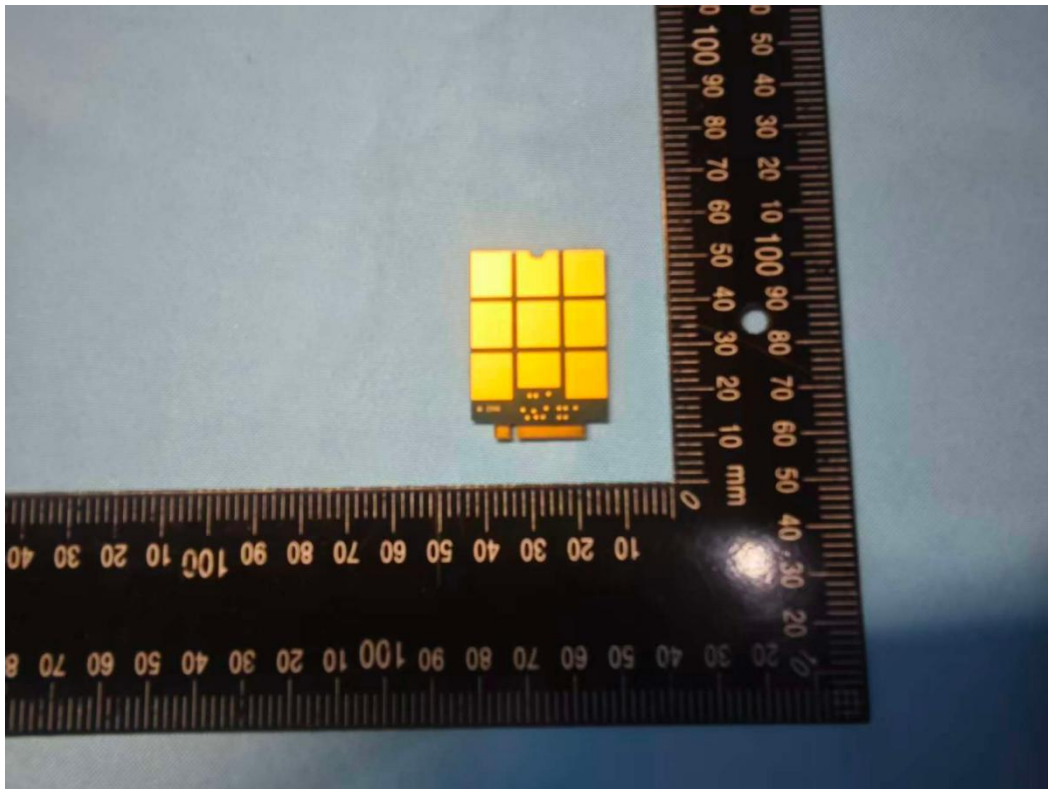
Photo 10 PCB1 Green Mainboard + LTE Module R62GT-V1.10
