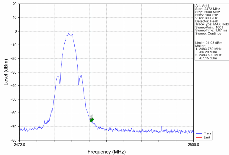
2M_HCH_2480MHz_Ant1_NTNV
