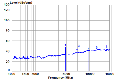
BLE_2M_TX_CH_19_Vertical-Avg
