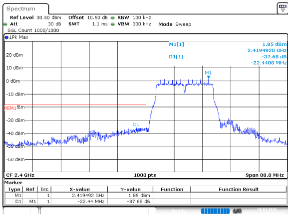
802.11n20_2412MHz
