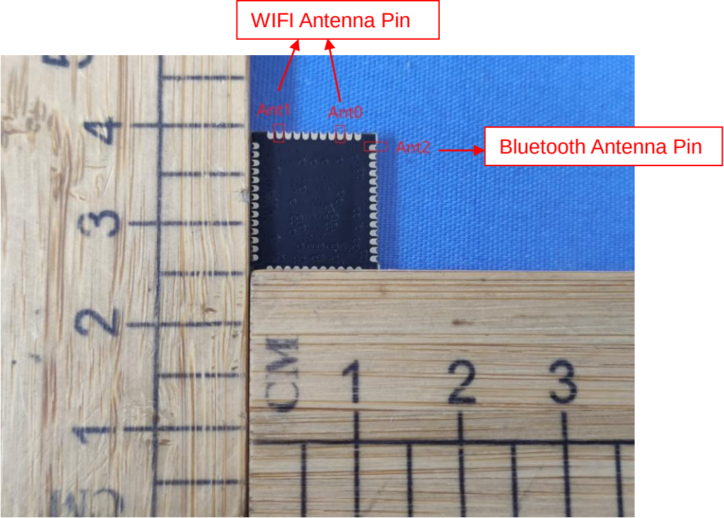
Antenna
