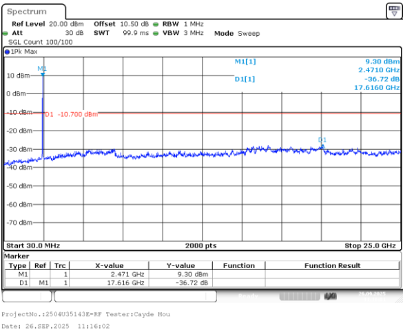
802.11n20_2462MHz_Chain 1
