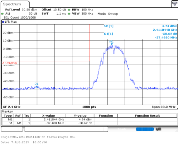
802.11b_2412MHz_Chain 0
