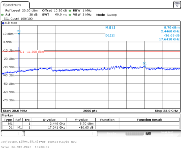
802.11n20_2437MHz_Chain 0
