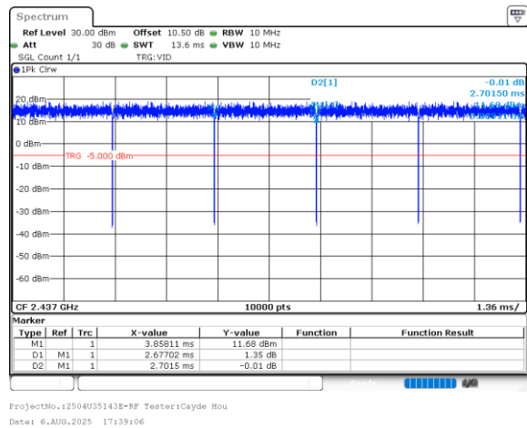
802.11n20_2437MHz_Chain 0
