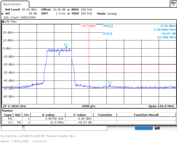
802.11n20_2462MHz_Chain 1
