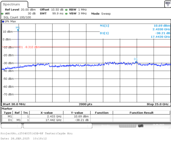
802.11b_2437MHz_Chain 0
