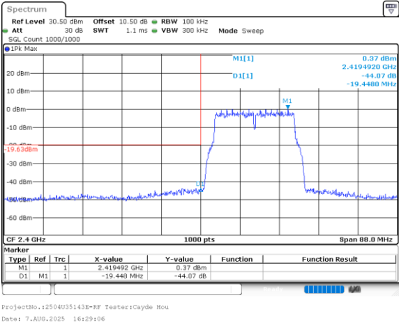
802.11n20_2412MHz_Chain 0
