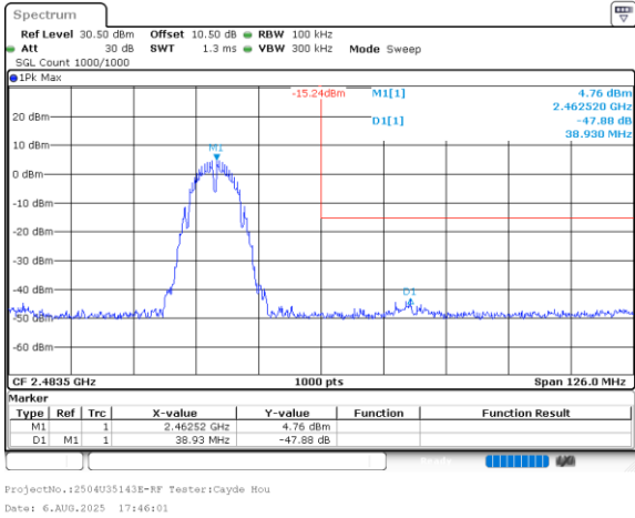
802.11b_2462MHz_Chain 0
