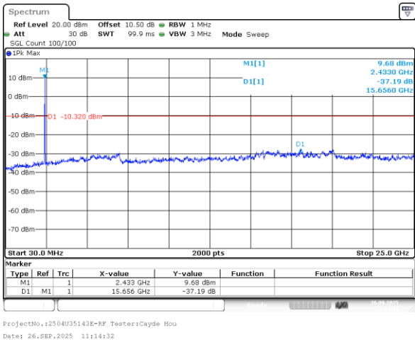
802.11n20_2437MHz_Chain 1
