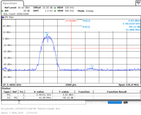
802.11b_2462MHz_Chain 1
