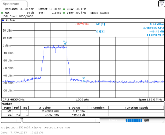
802.11n20_2462MHz_Chain 0
