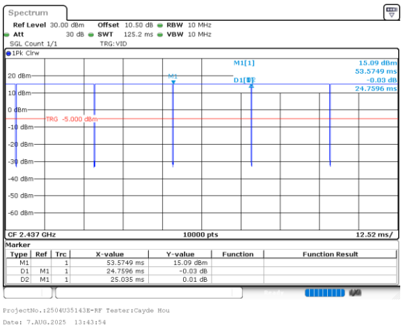
802.11b_2437MHz_Chain 1
