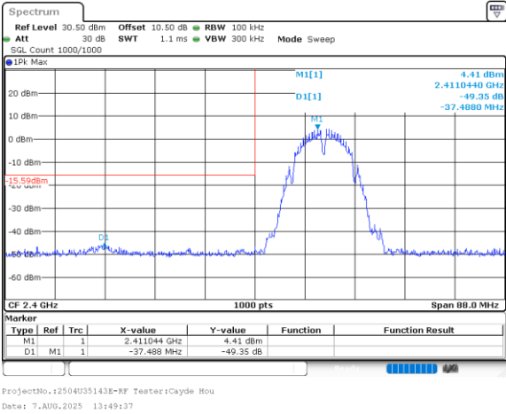
802.11b_2412MHz_Chain 1
