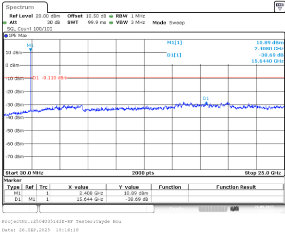
802.11b_2412MHz_Chain 0
