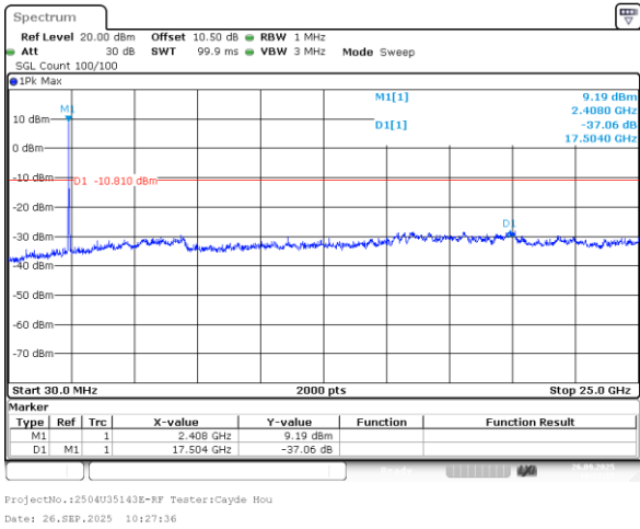
802.11n20_2412MHz_Chain 0
