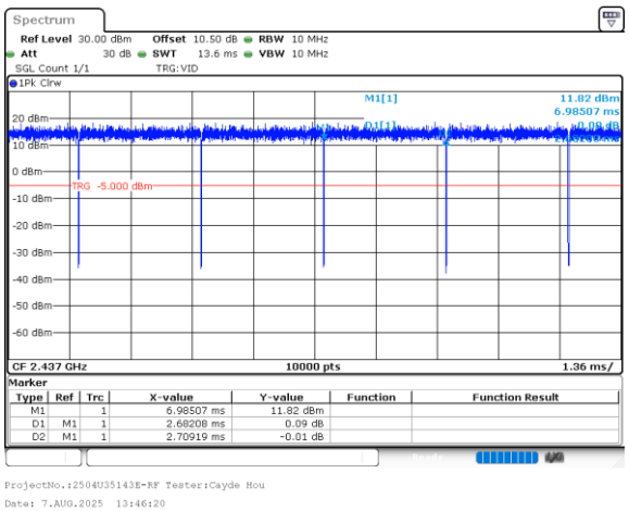
802.11n20_2437MHz_Chain 1
