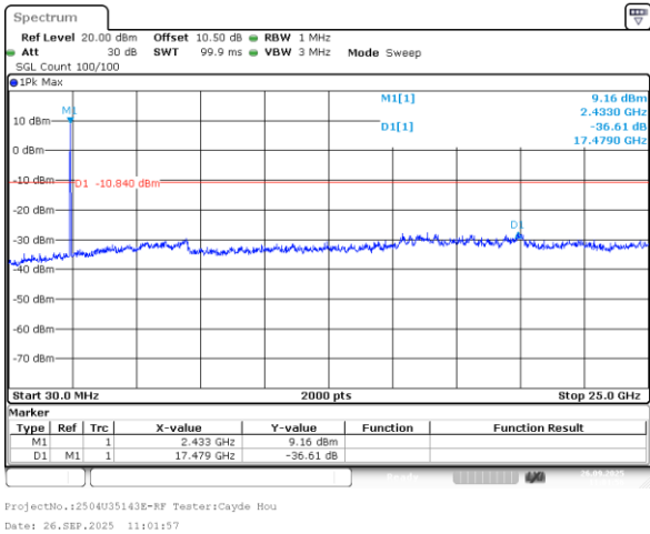
802.11b_2437MHz_Chain 1
