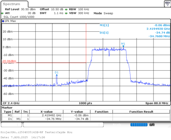
802.11n20_2412MHz_Chain 1
