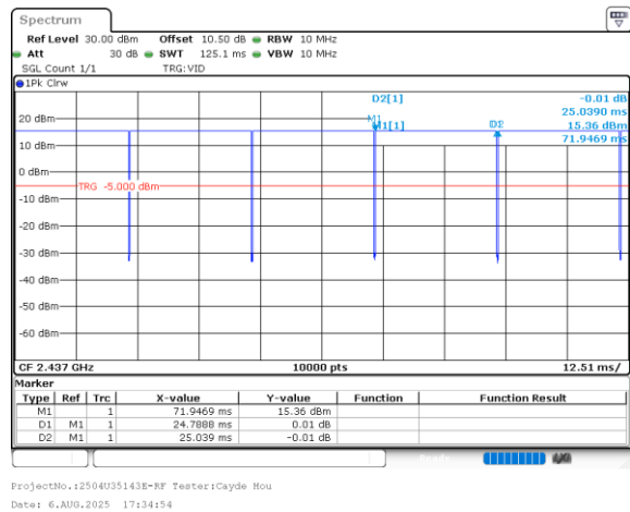
802.11b_2437MHz_Chain 0
