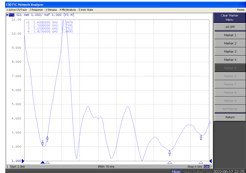
VSWR
