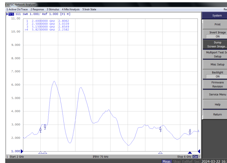
VSWR
