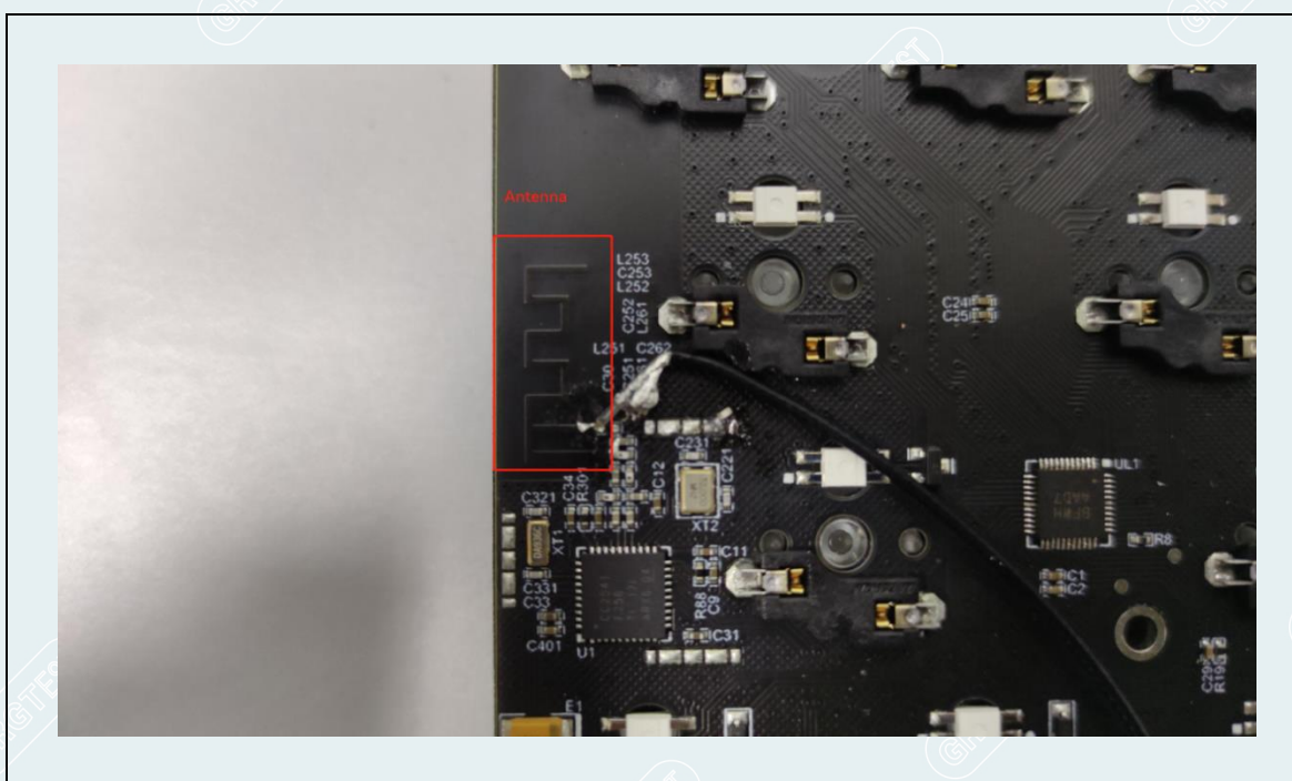
Antenna
